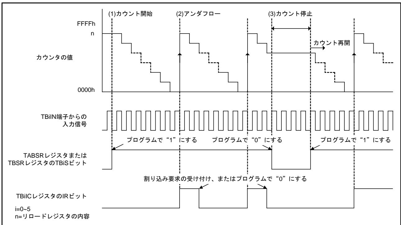
図 3.1 イベントカウンタモードの動作
