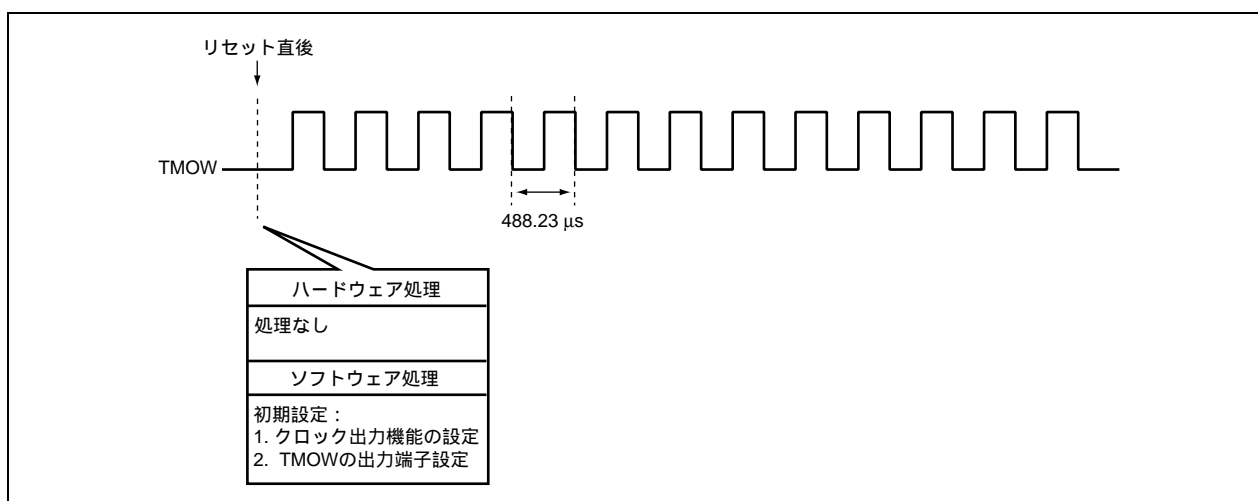
図 3.1 タイマ A クロック出力機能によるクロック出力の動作原理
