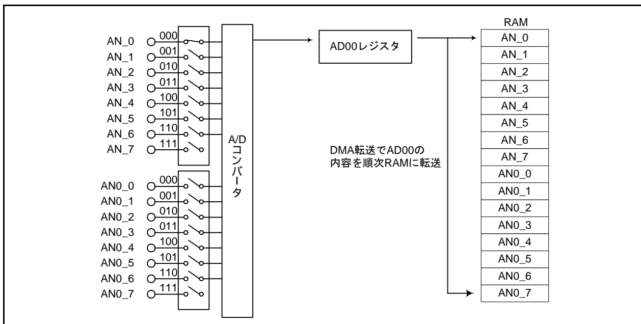
図 3.1 マルチポート単掃引モードの動作例
