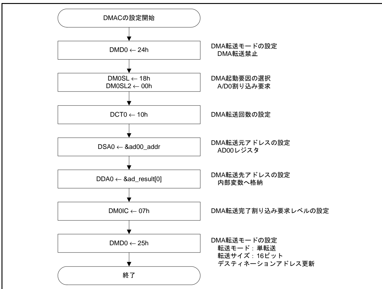
図 3.3 マルチポート単掃引モードの設定手順 (2/2)
