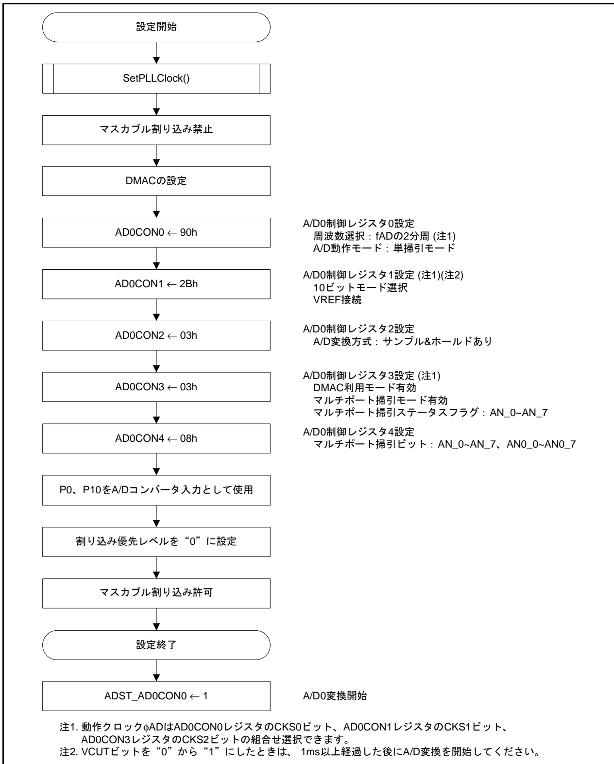
図 3.2 マルチポート単掃引モードの設定手順 (1/2)
