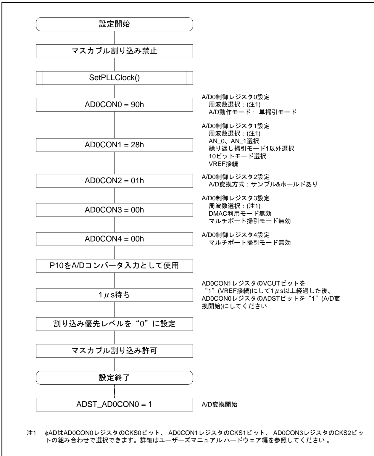
図 3.2 単掃引モードの設定手順
