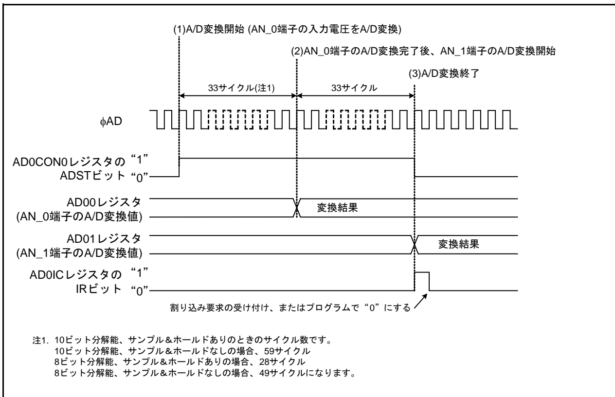
図 3.1 単掃引モードの動作例
