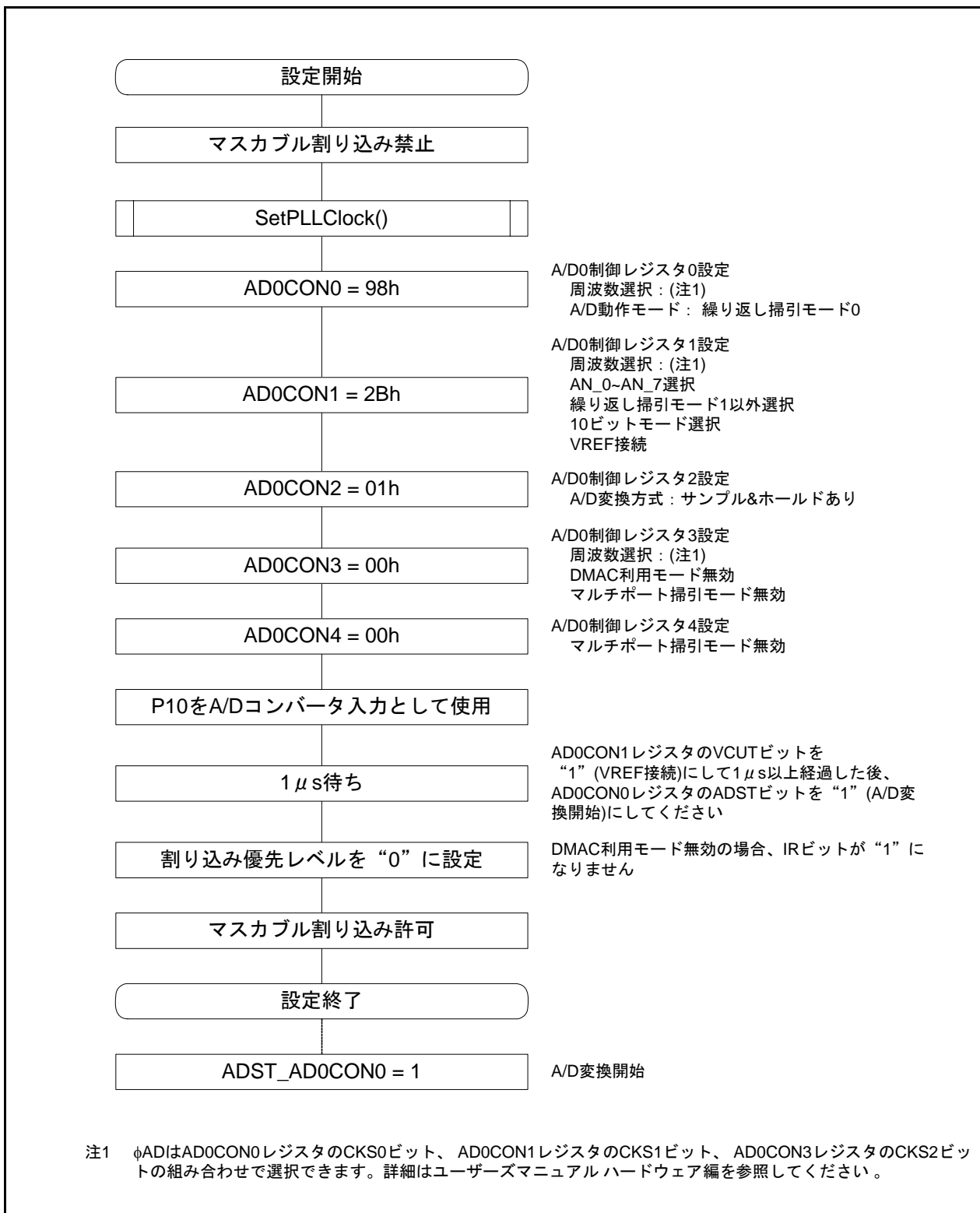
図 3.2 繰り返し掃引モード0の設定手順
