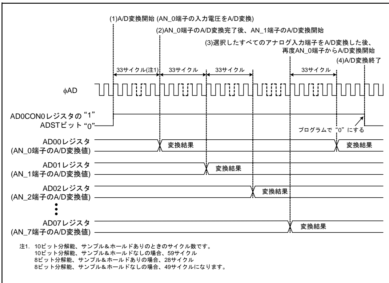
図 3.1 繰り返し掃引モード0の動作例
