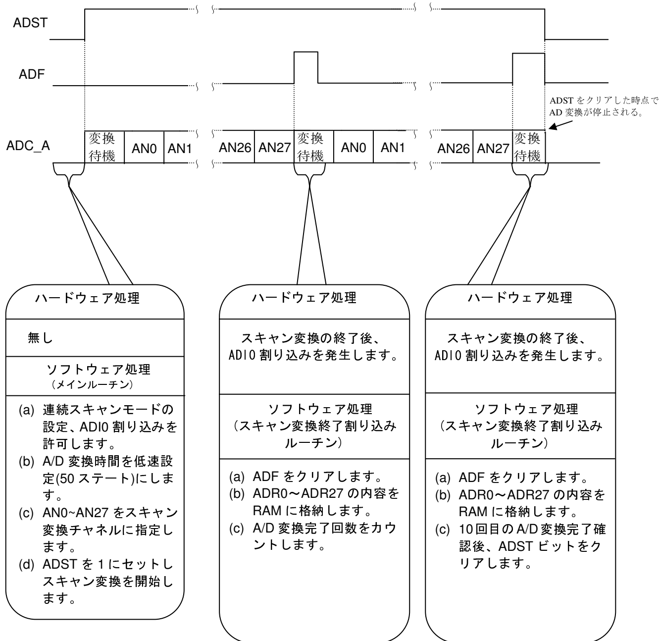
図 2 A/D 変換動作説明
