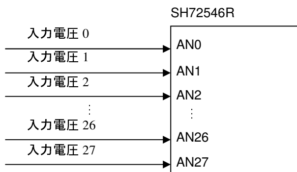
図 1 SH72546R による電圧の測定ブロック図
