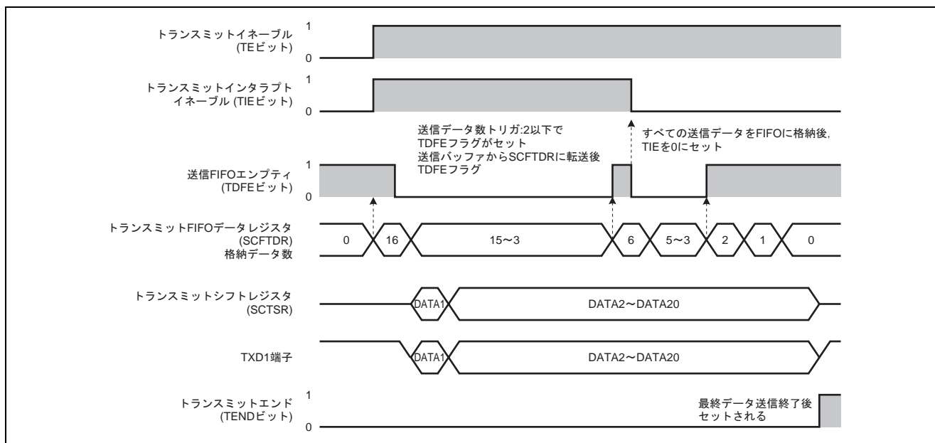
図3 送信動作
