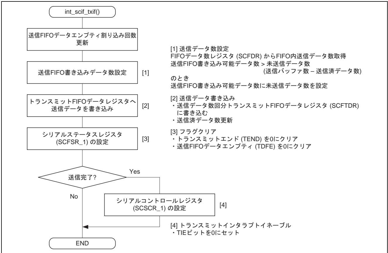
図 8 SCIF 送信 FIFO データエンプティ割り込み関数の処理フロー
