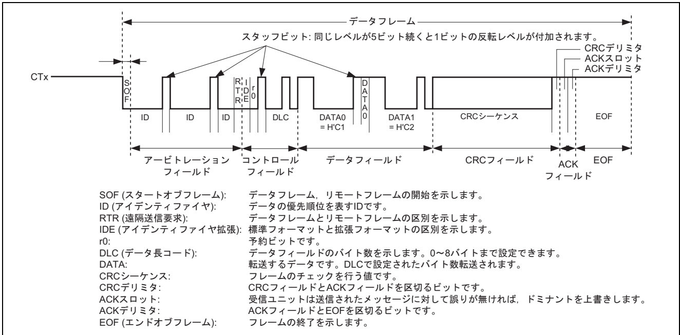
図 5 データフレームの送信波形
