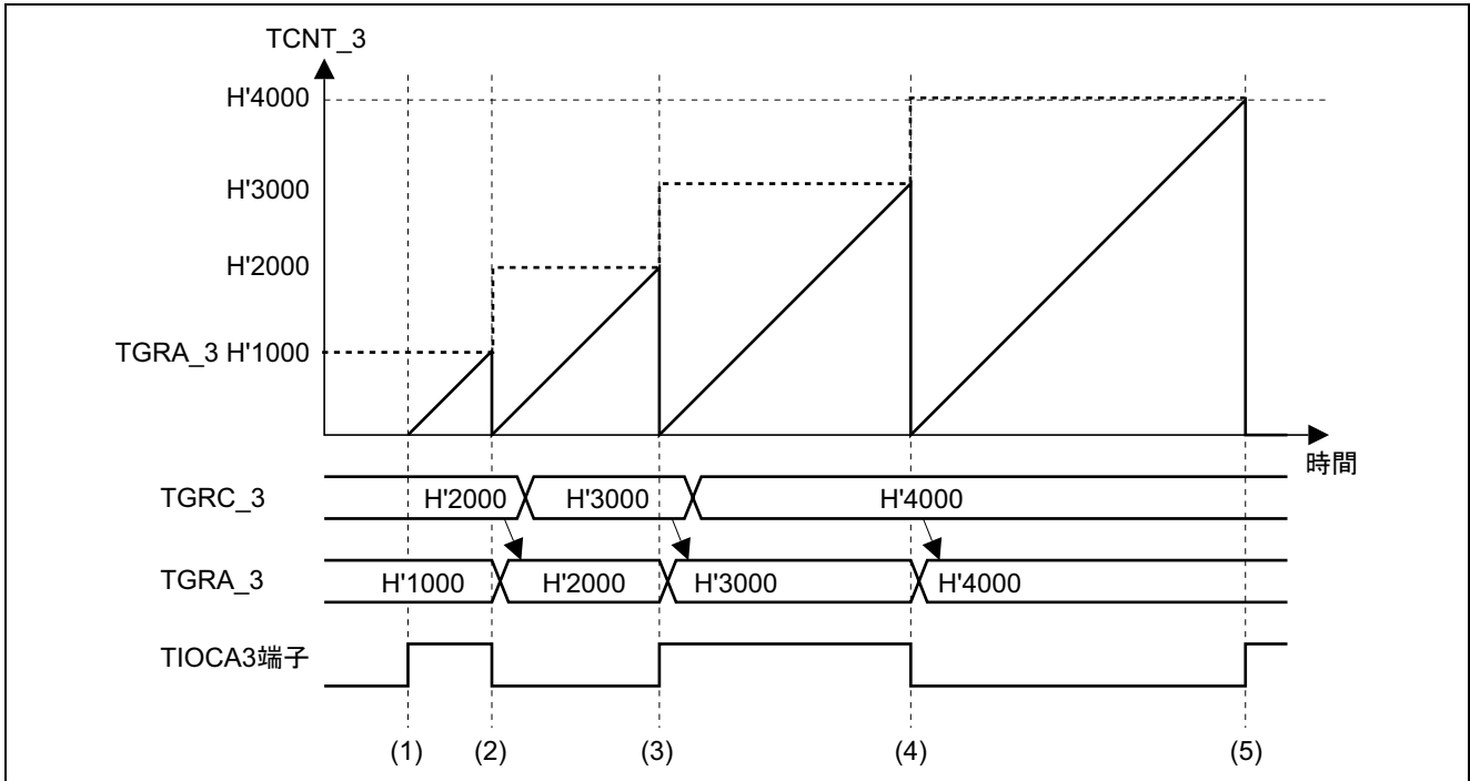
図2 パルス出力動作説明
