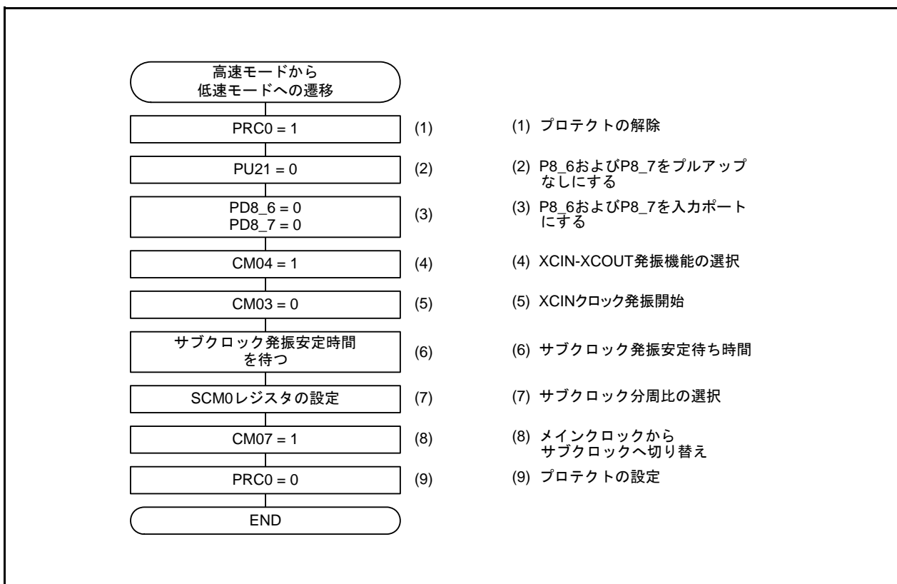
図3.2 高速モードから低速モードへの遷移
