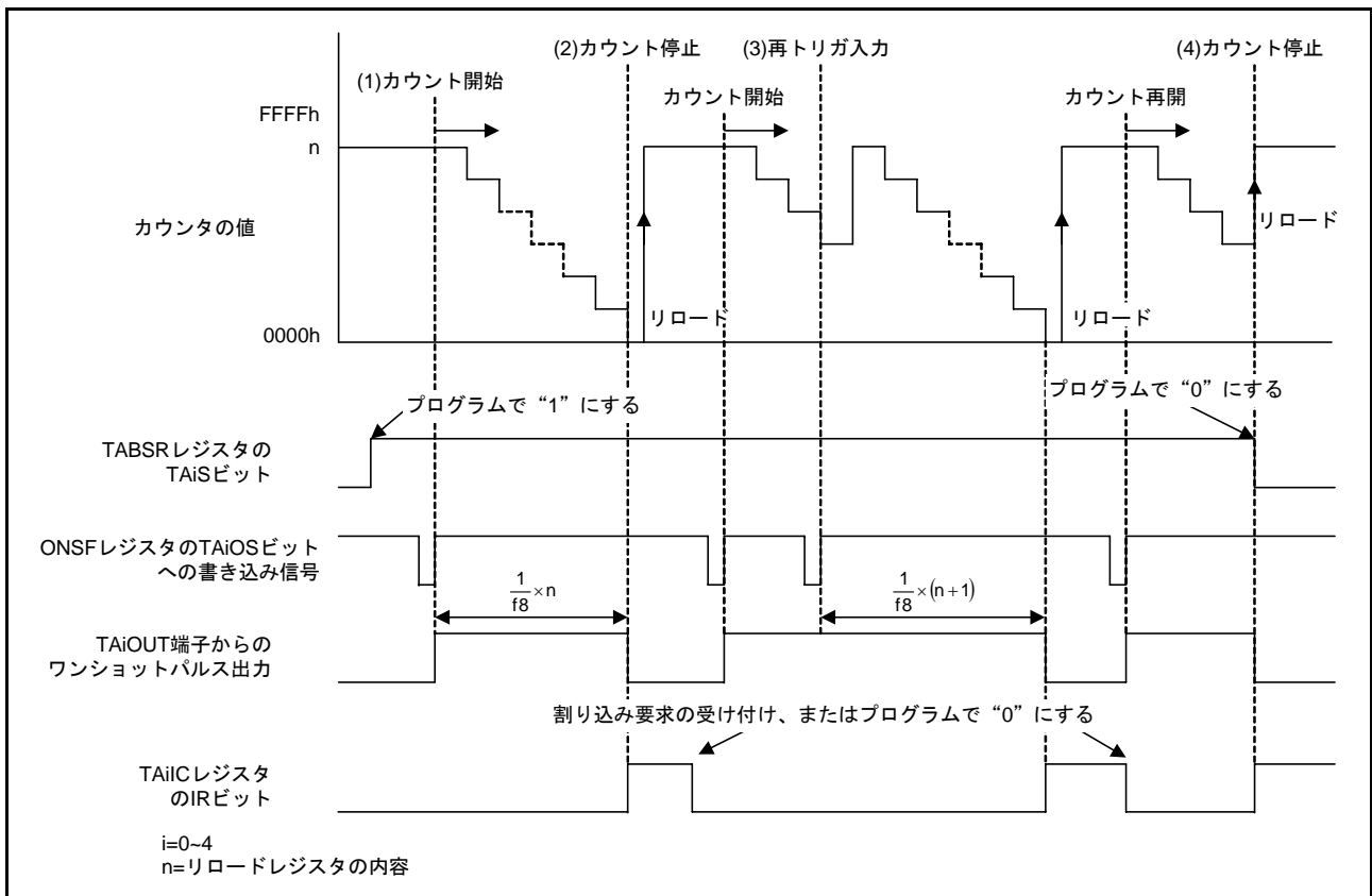
図 3.1 ワンショットタイマモードの動作
