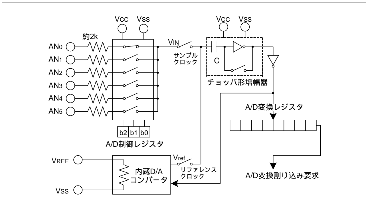
図 3.1 A/Dコンバータ等価回路
