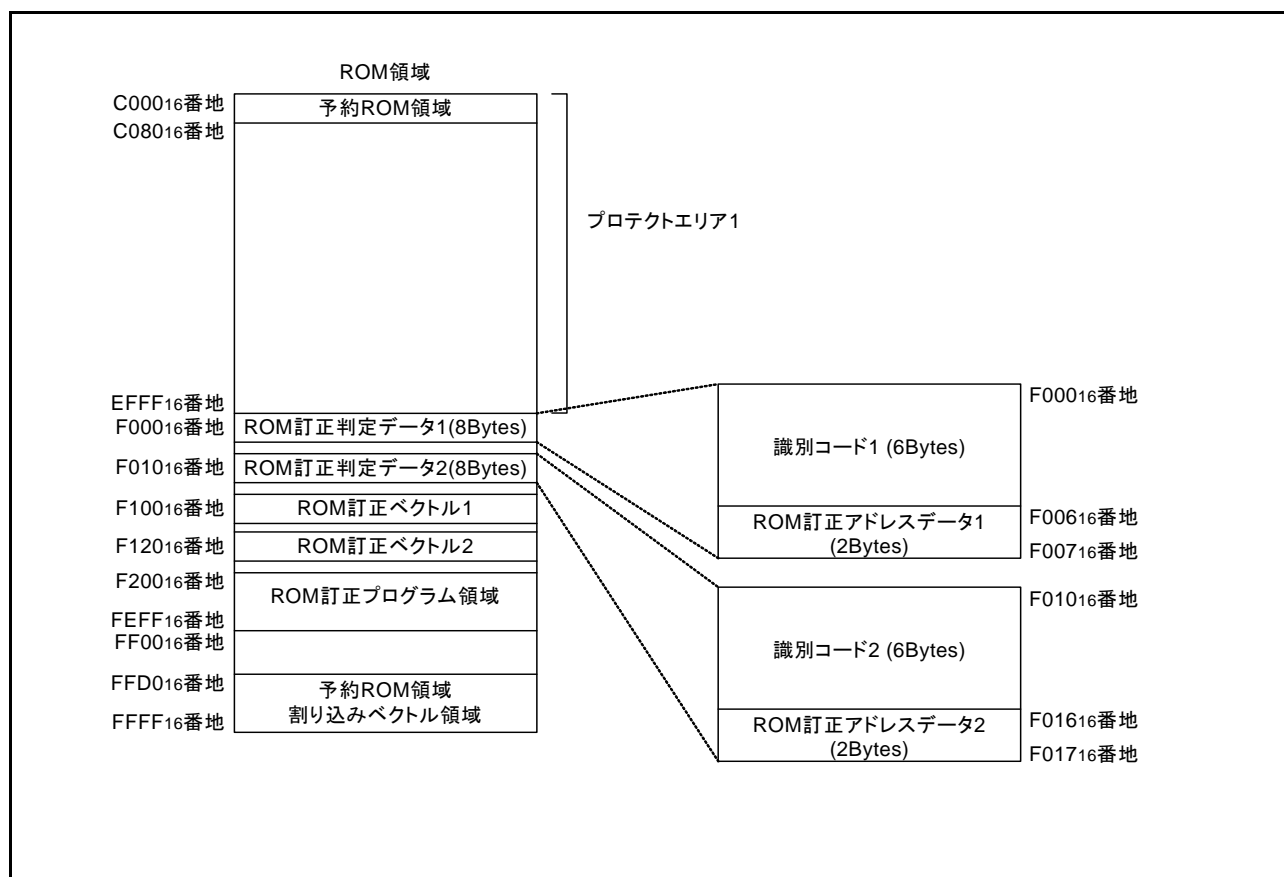
図 3.4 M38D24G4 の場合の ROM マップ
