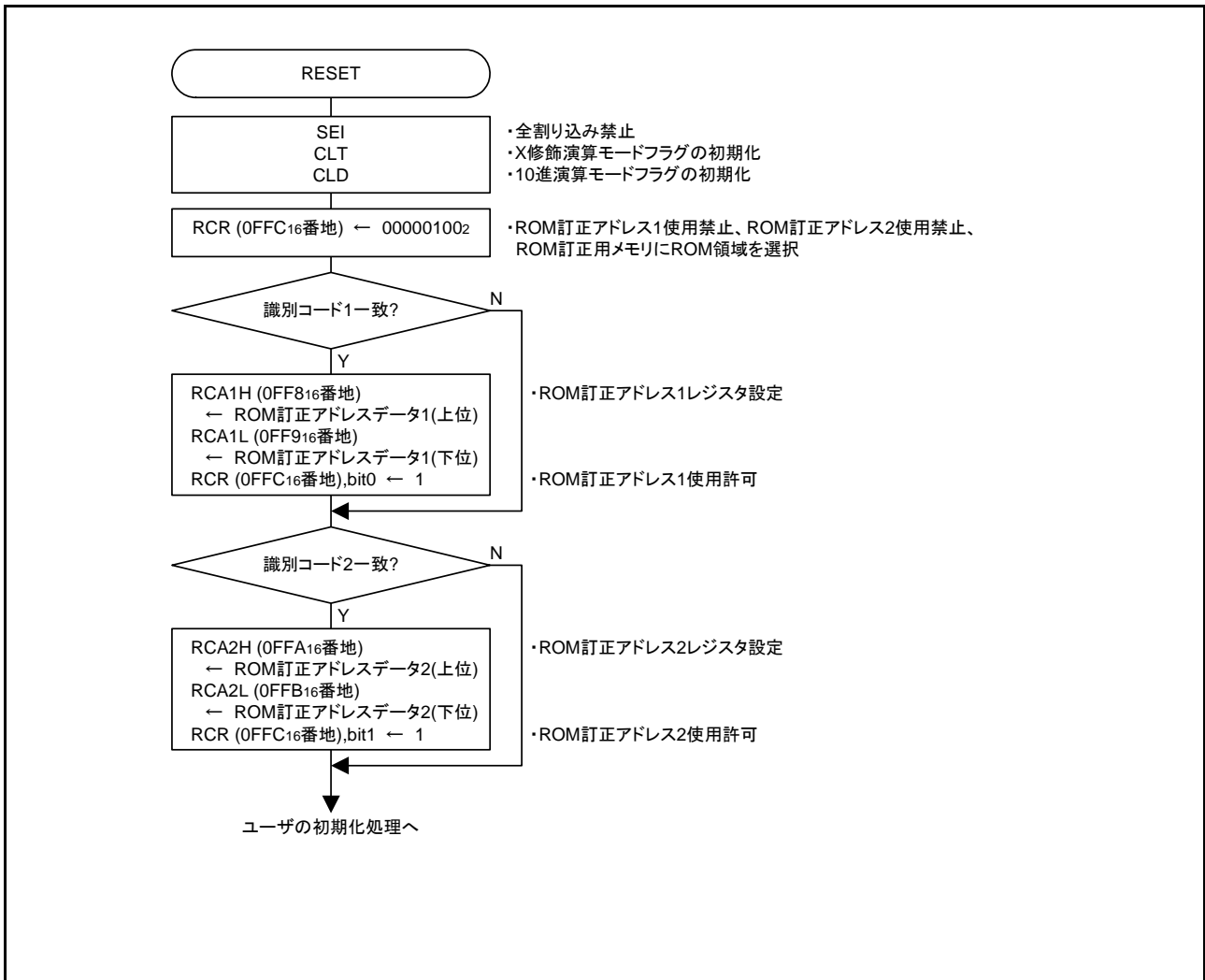
図 3.5 スタートアップ処理の制御手順
