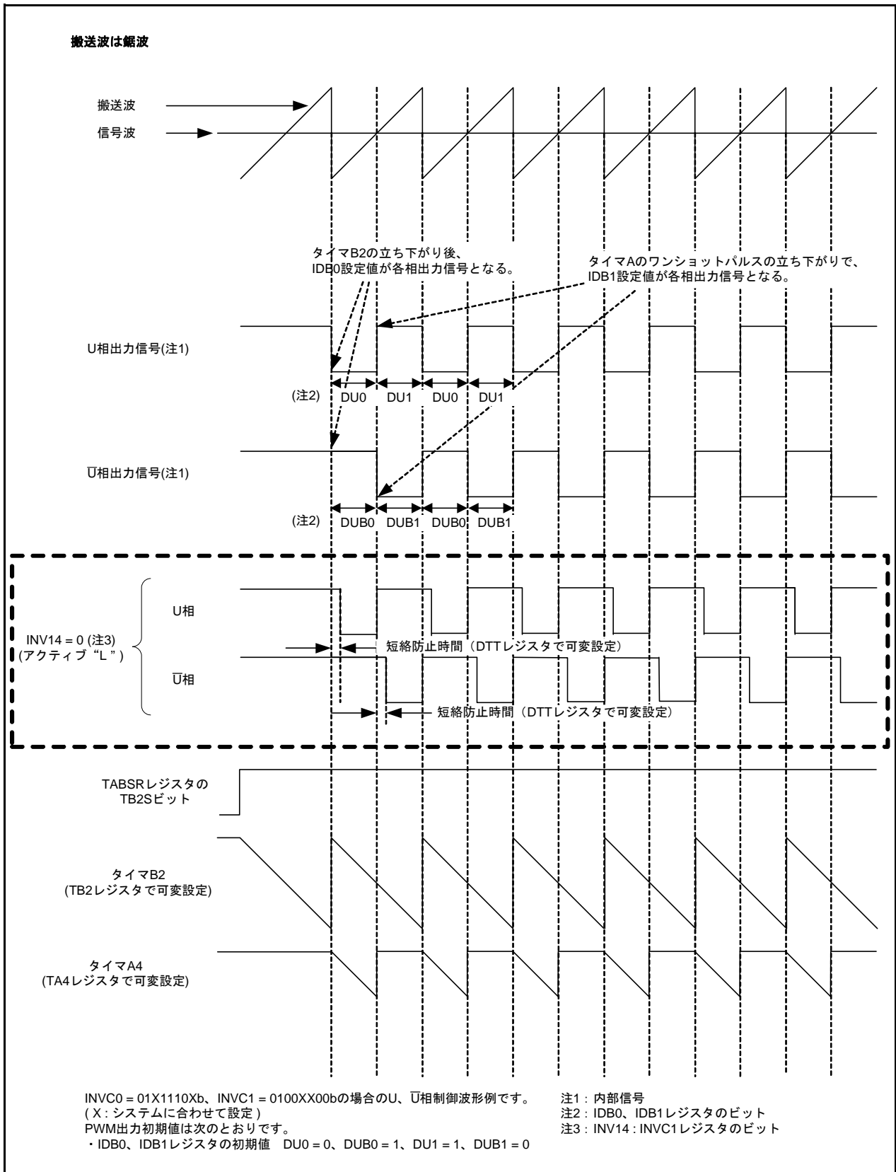
図 3.1 鋸波変調動作タイミング
