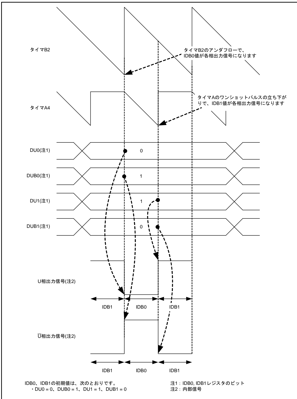
図 3.3 U相出力信号の動作例
