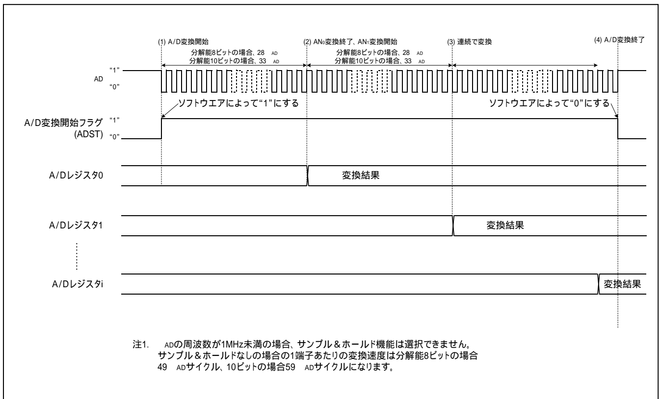
図 1 繰り返し掃引モード 0 の動作タイミング
