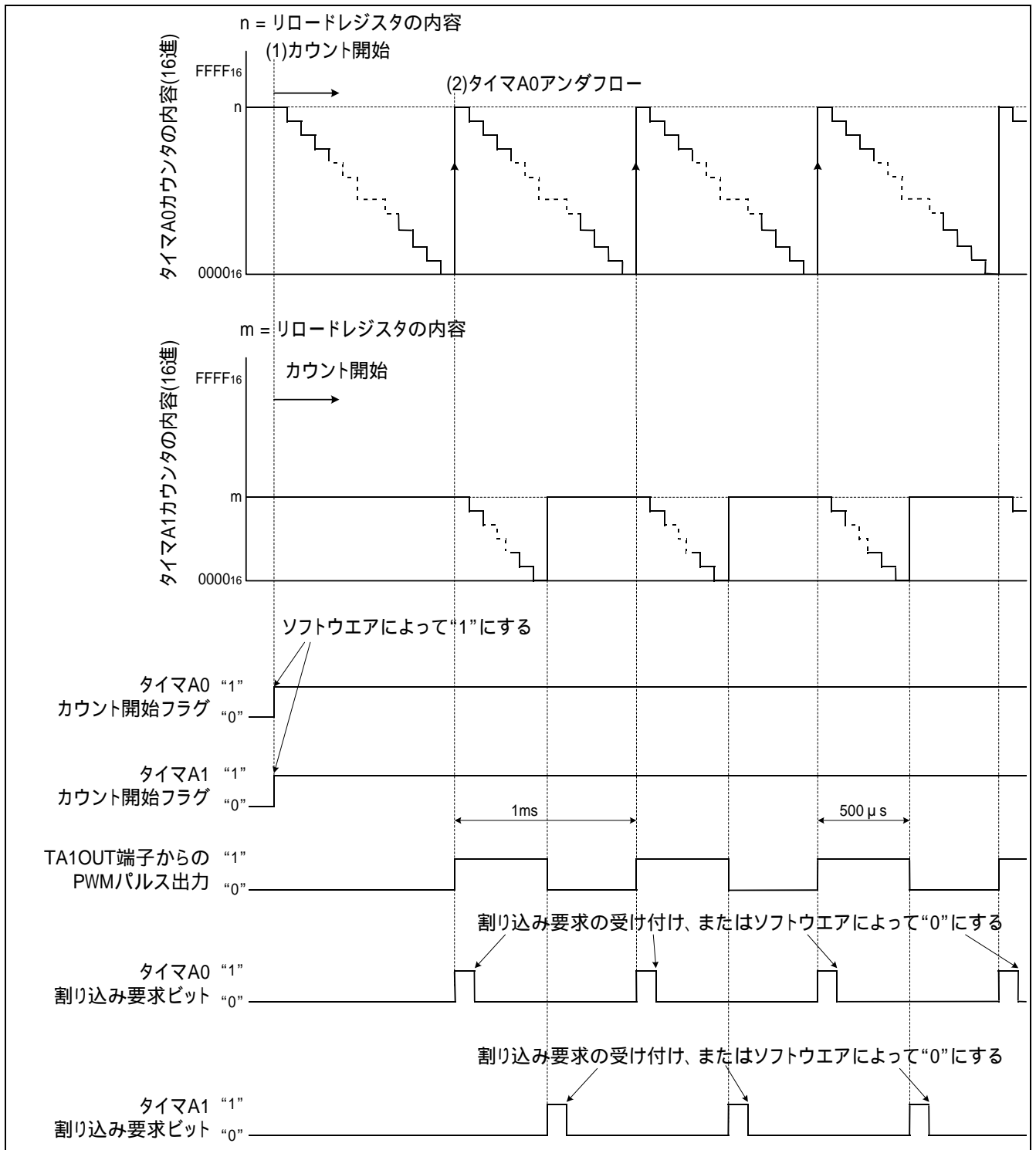
図 1 周期およびデューティ可変のPWM 出力の動作タイミング
