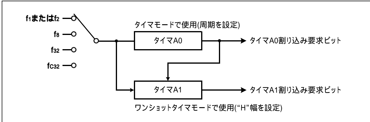
図 2 周期およびデューティ可変の PWM 出力のタイマ接続図
