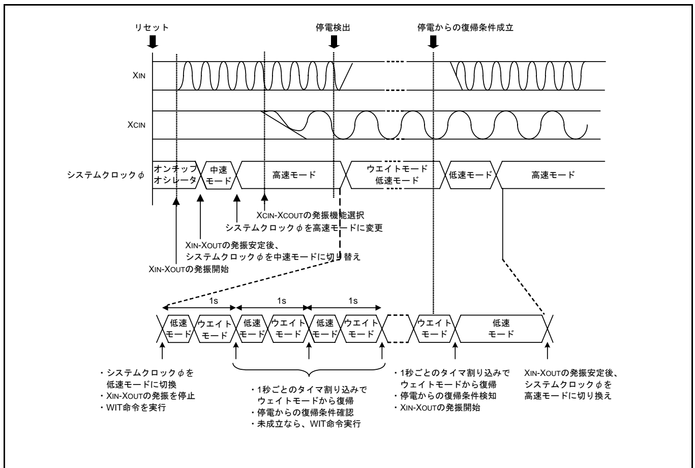
図 3.1 停電時のシステムクロックφのモード移行例
