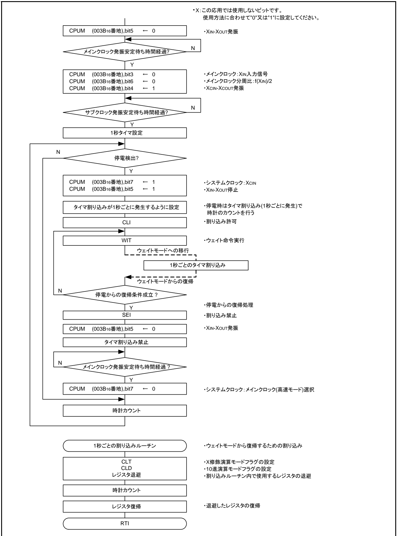
図 3.3 制御手順
