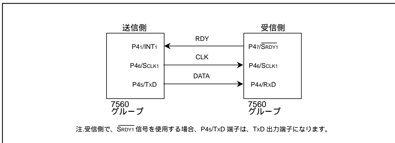
図 3.1 接続図
