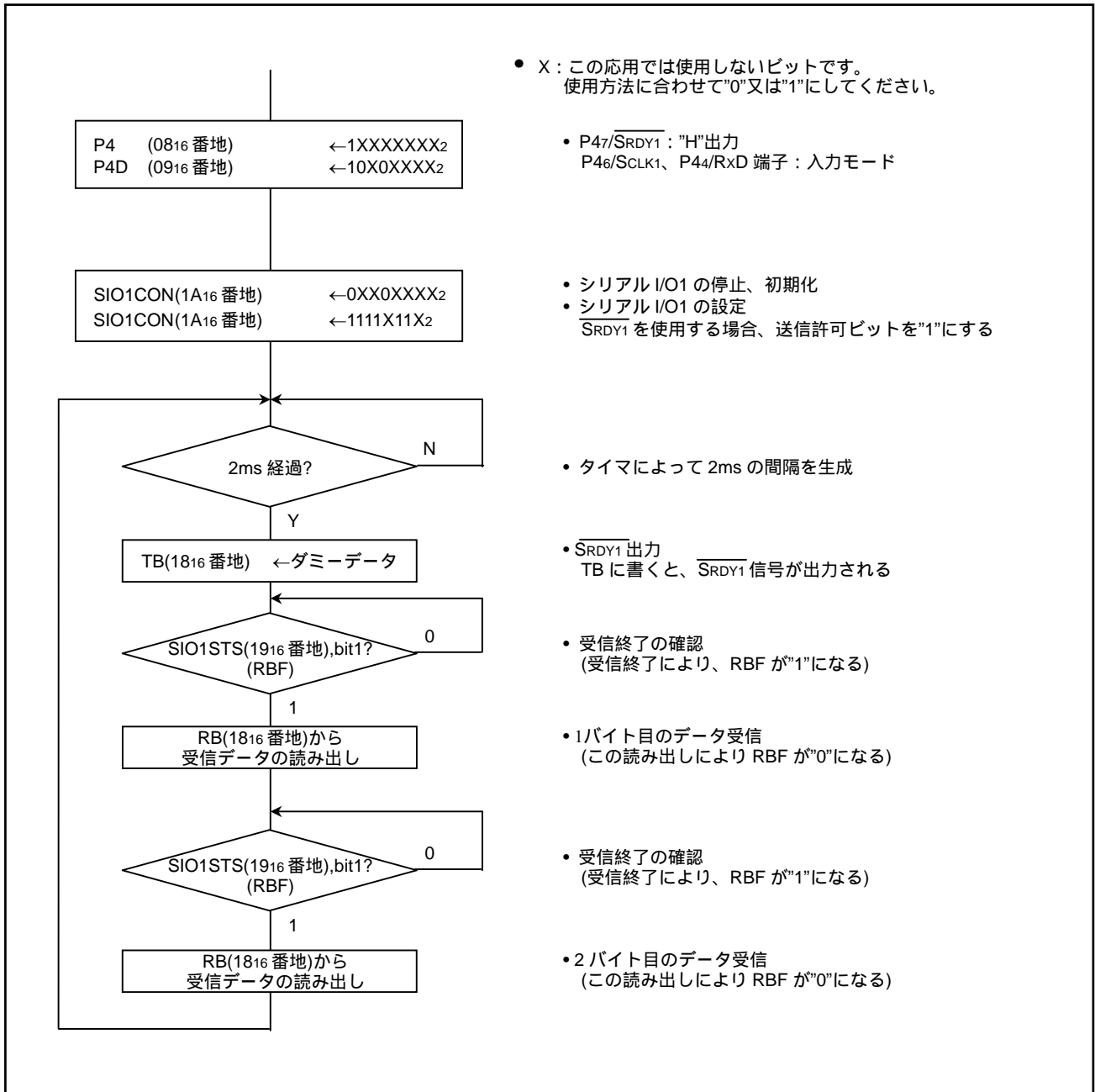
図 3.6 受信側の制御手順
