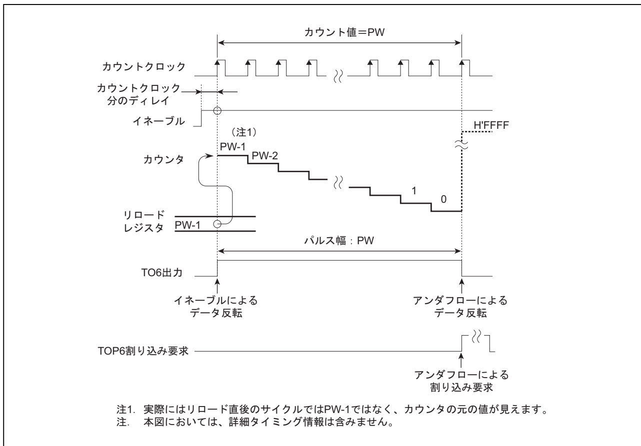
図 4.5.1 TOP ワンショットパルス出力タイミング図
