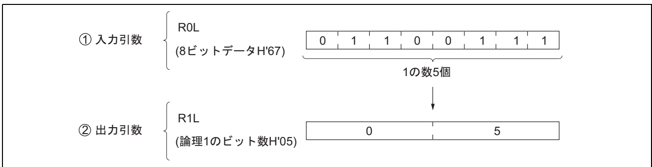
図 9-1 ソフトウェア HCNT の実行例
