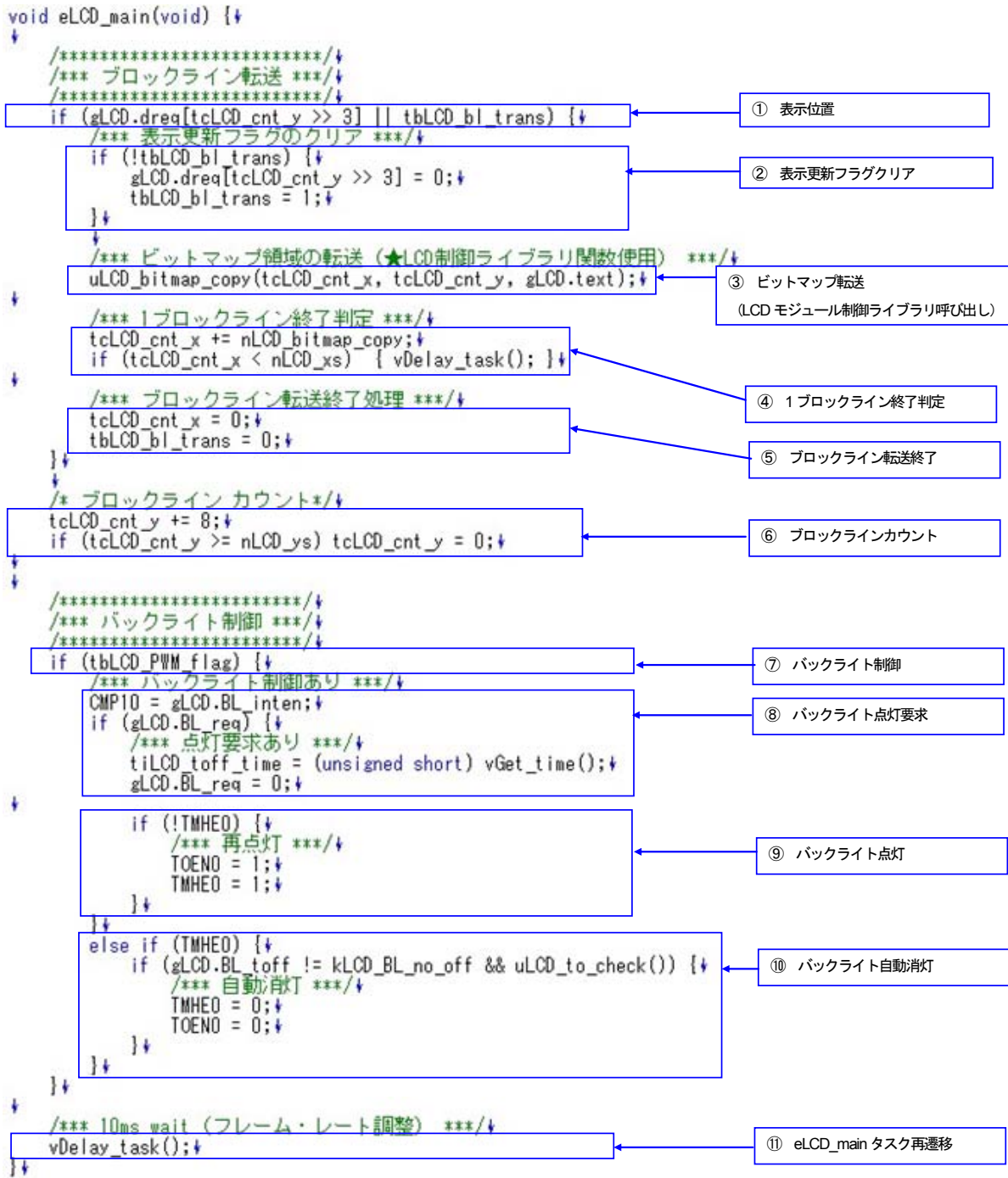
図3 - 14 eLCD_main関数プログラム・リスト
