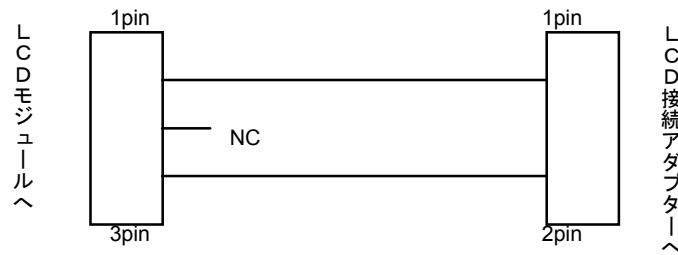
図2 - 39 WG240128D 接続ハーネス図 (バックライト用)
