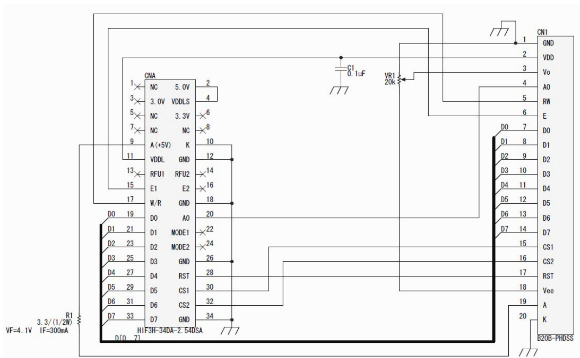
図2 - 16 SG12864C LCD接続アダプタ回路図
