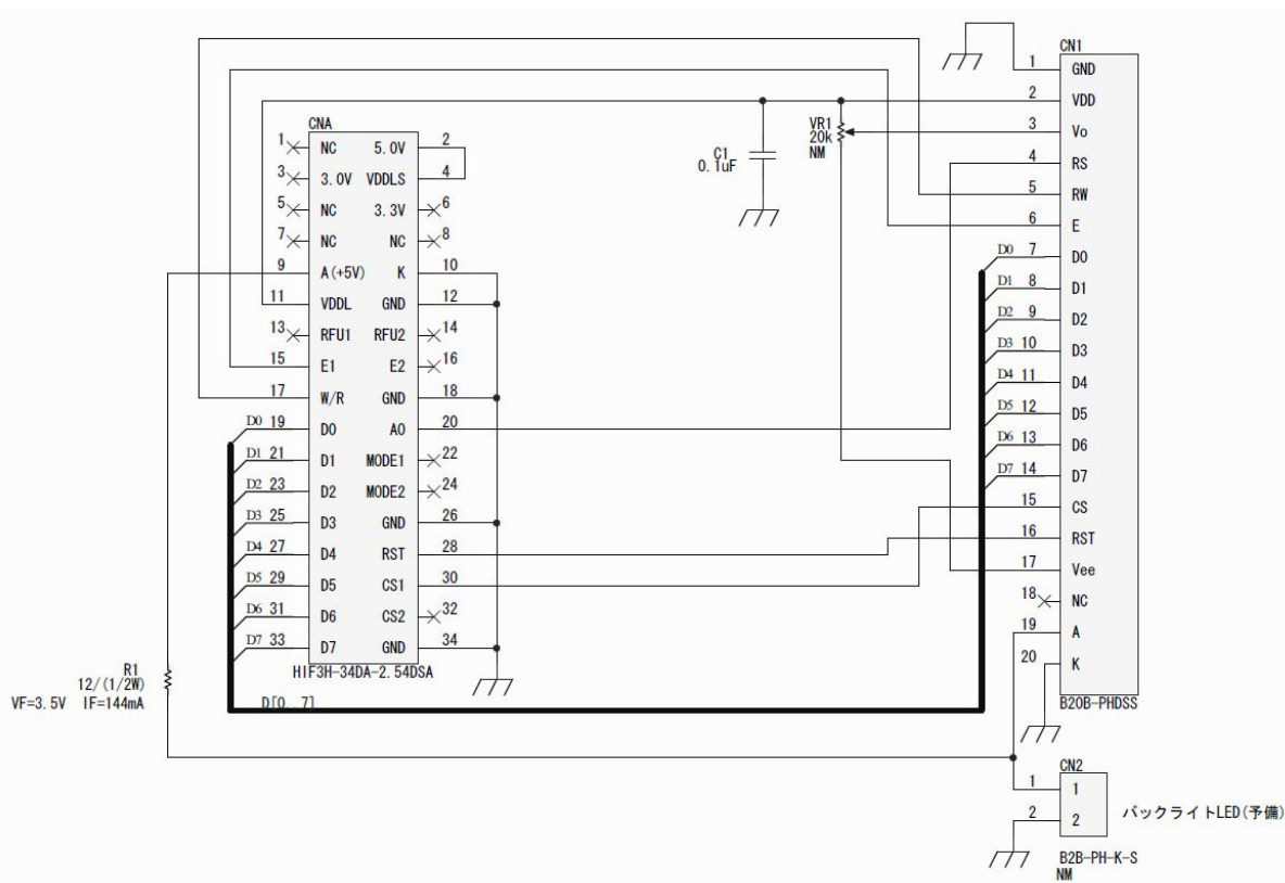
図2 - 37 WG240128D LCD接続アダプタ回路図
