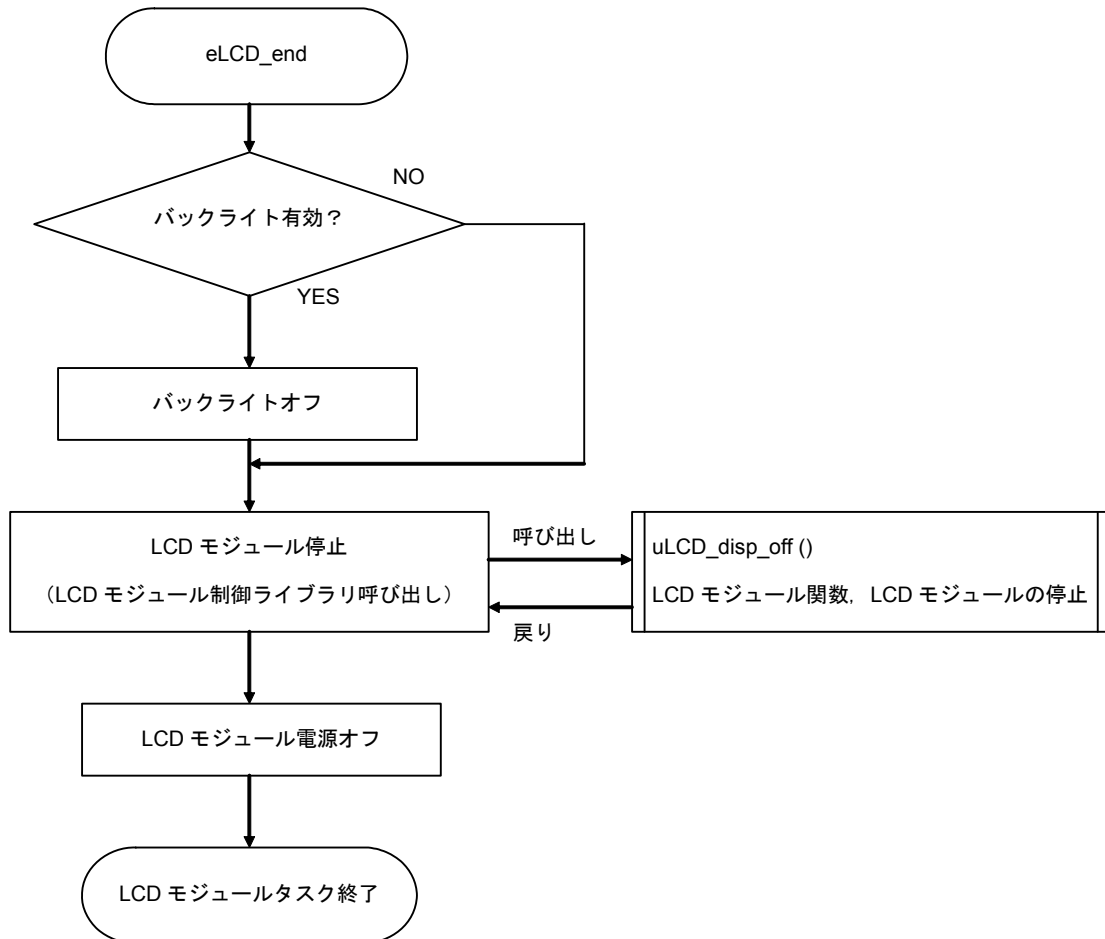
図3 - 15 eLCD_main関数フローチャート
