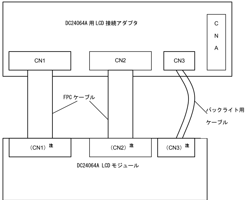
図2 - 11 DC24064A 接続図
