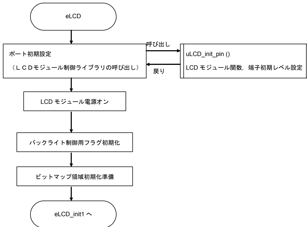
図3 - 5 eLCD関数フローチャート
