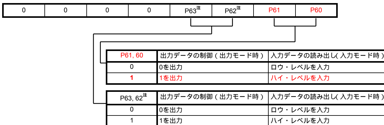
図4 - 7 ポート・レジスタ6 (P6) のフォーマット
