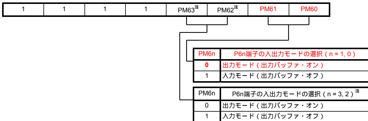
図4 - 8 ポート・モード・レジスタ6 (PM6) のフォーマット
