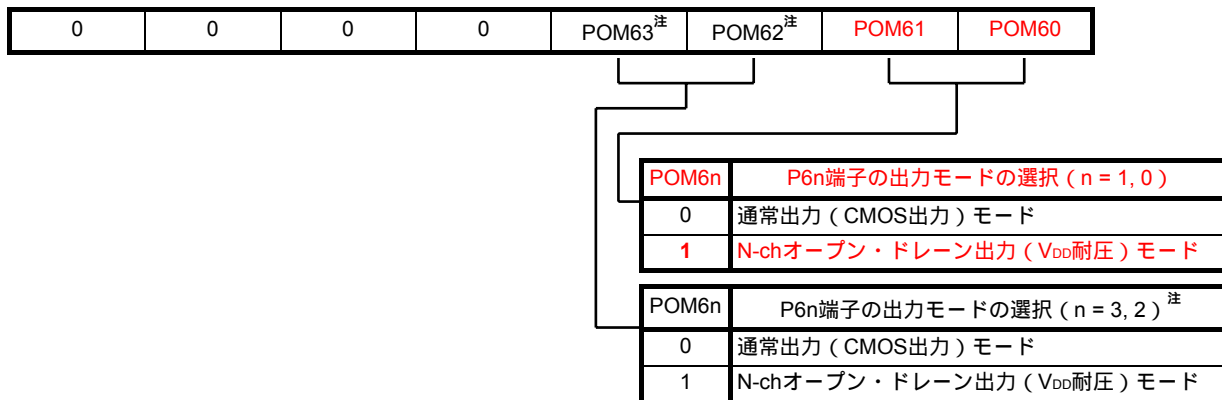
図4 - 6 ポート出力モード・レジスタ6 (POM6) のフォーマット
