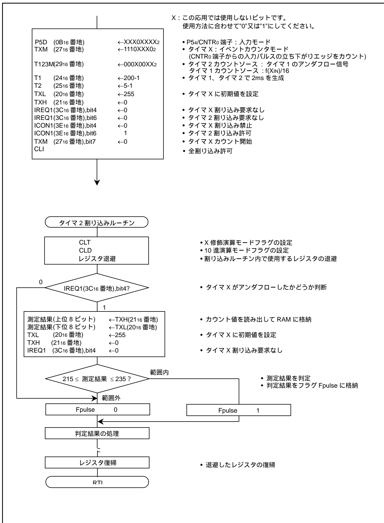
図 3.3 制御手順
