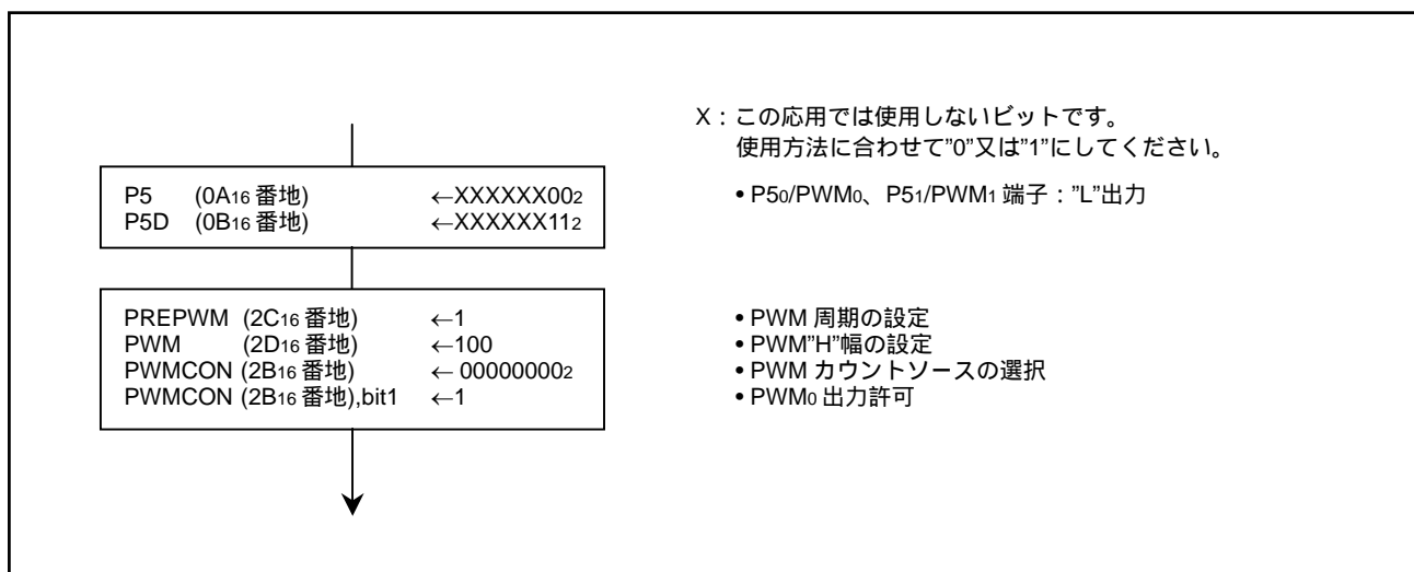
図 3.4 制御手順
