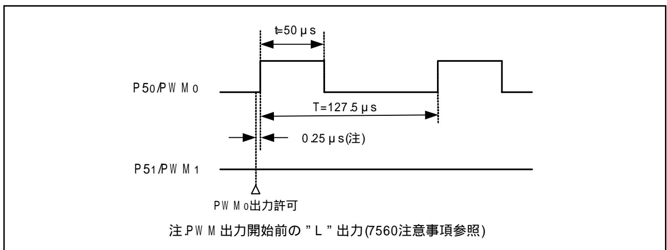
図 3.2 PWM 出力タイミング図
