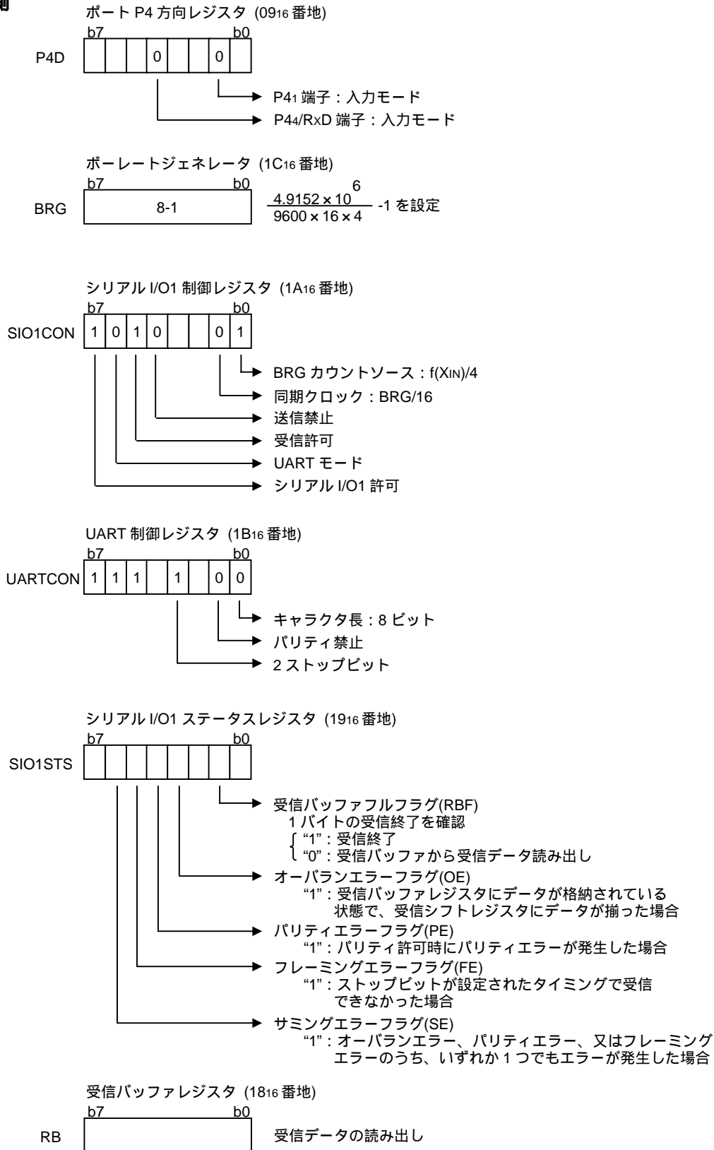
図 3.4 受信側関連レジスタの設定
