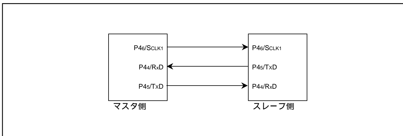
図 3.1 接続図
