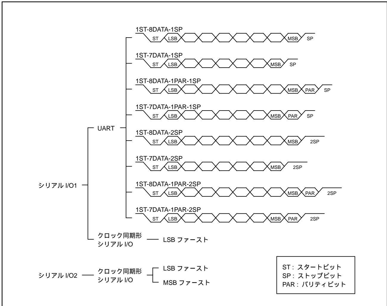
図 3.3 シリアル I/O 転送データフォーマット
