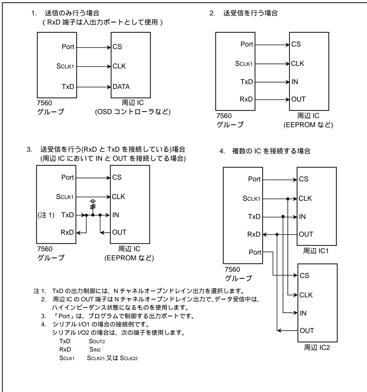
図 3.1 シリアル I/O の接続例 1
