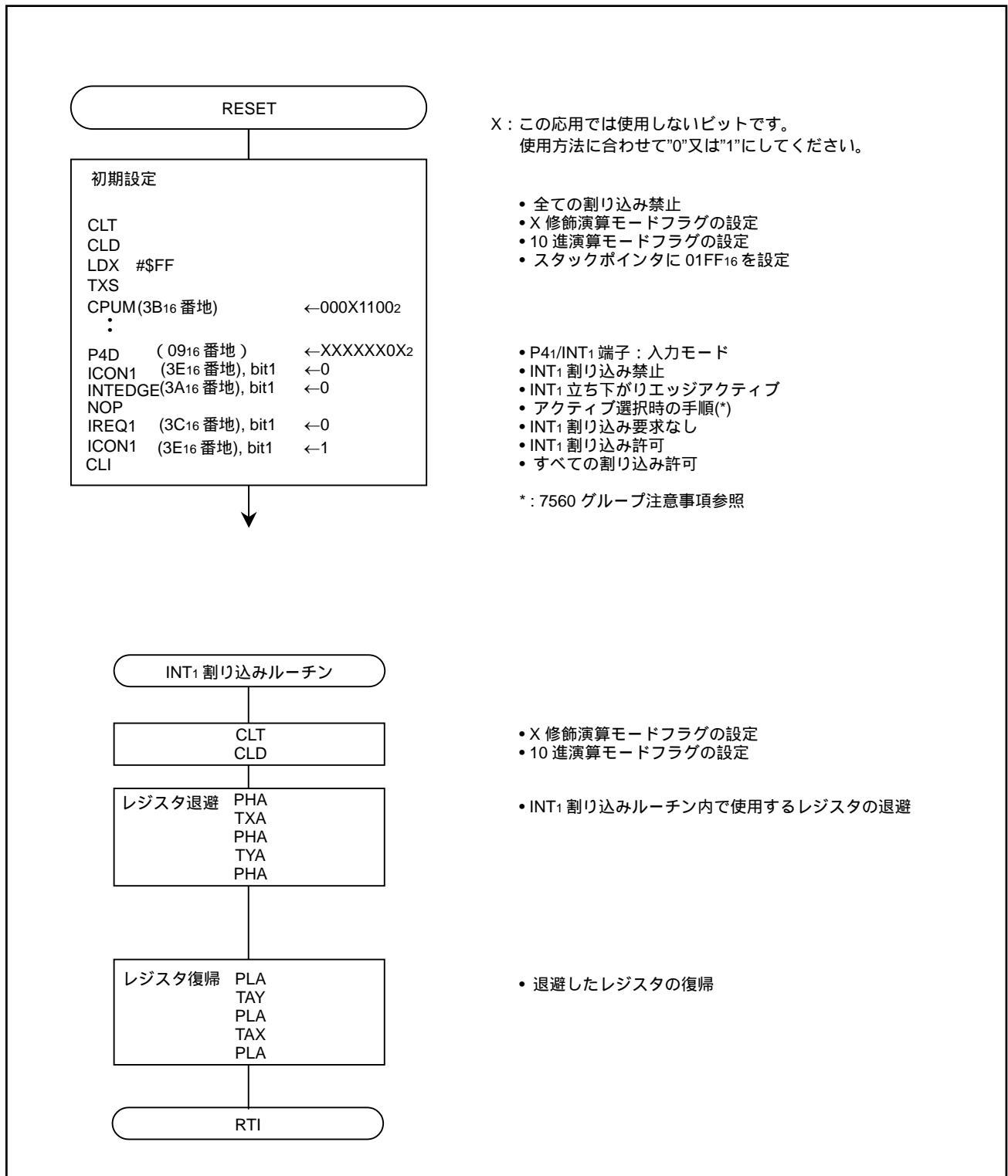
図 3.3 制御手順
