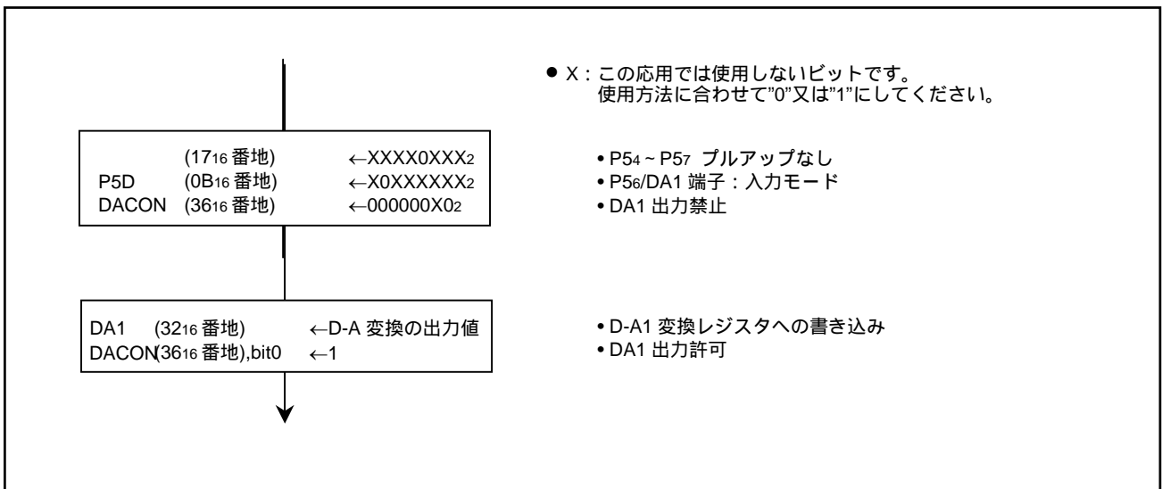
図 3.3 制御手順
