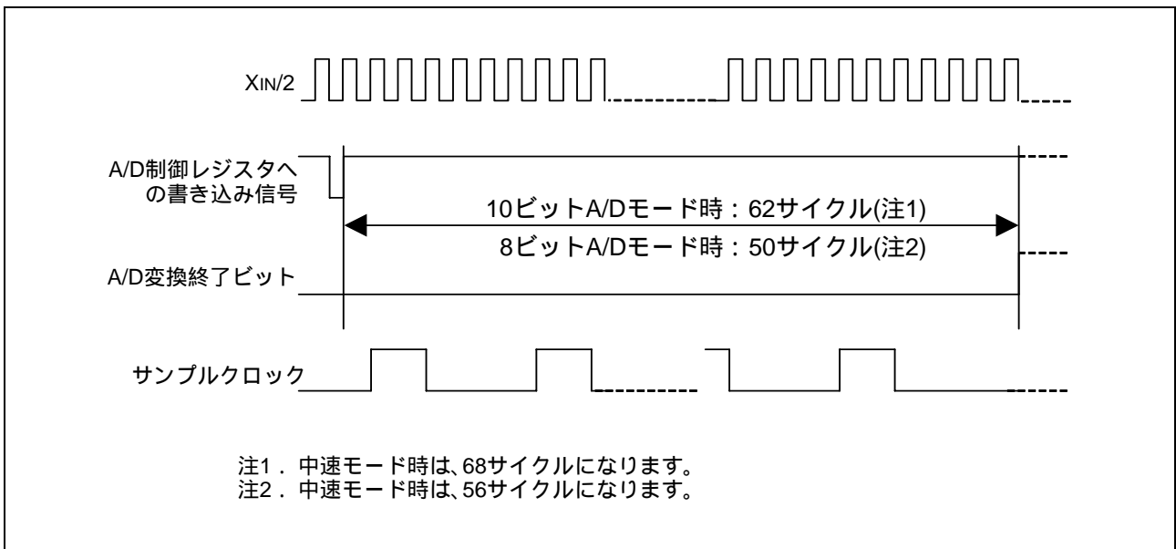
図 3.3 A/D変換タイミングチャート
