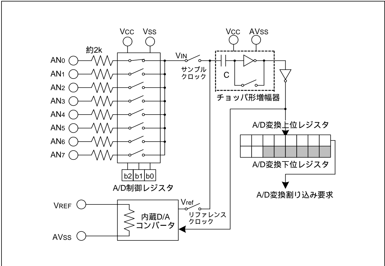
図 3.2 A/Dコンバータ等価回路
