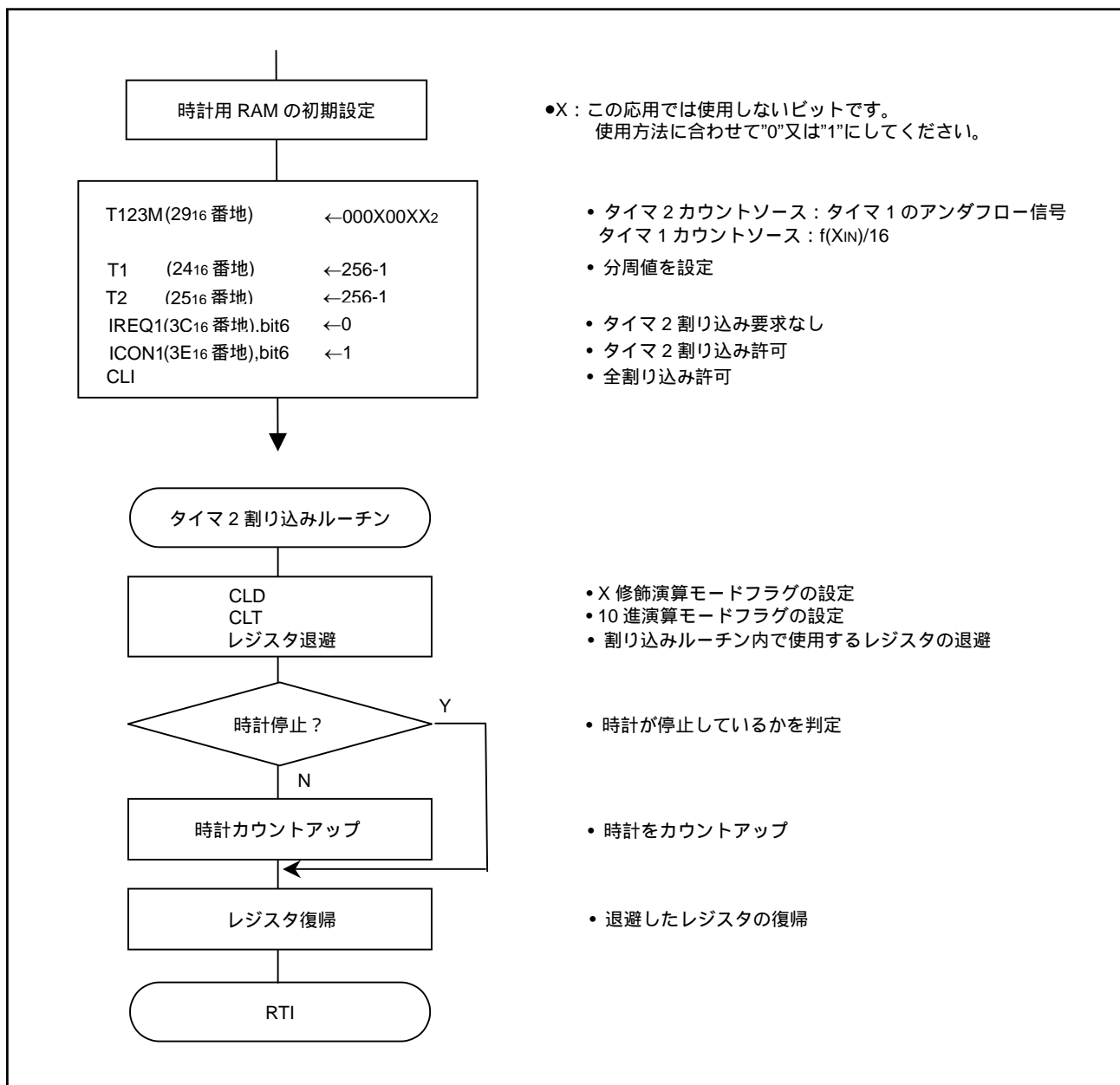
図 3.3 制御手順
