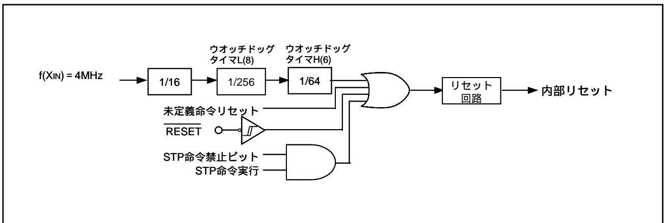
図 3.1 ウオッチドッグタイマの接続と分周比の設定
