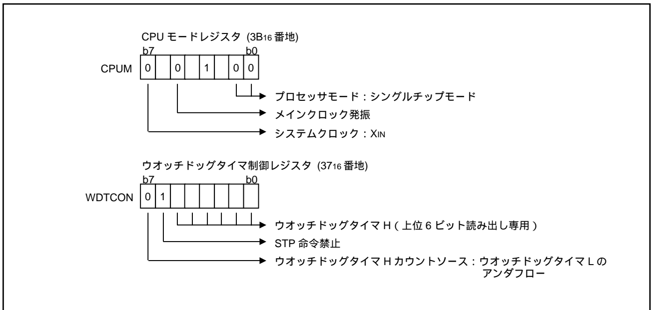
図 3.2 関連レジスタの設定
