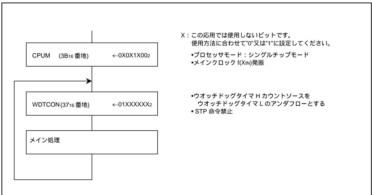
図 3.3 制御手順
