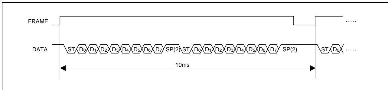
図 3.2 タイミング図
