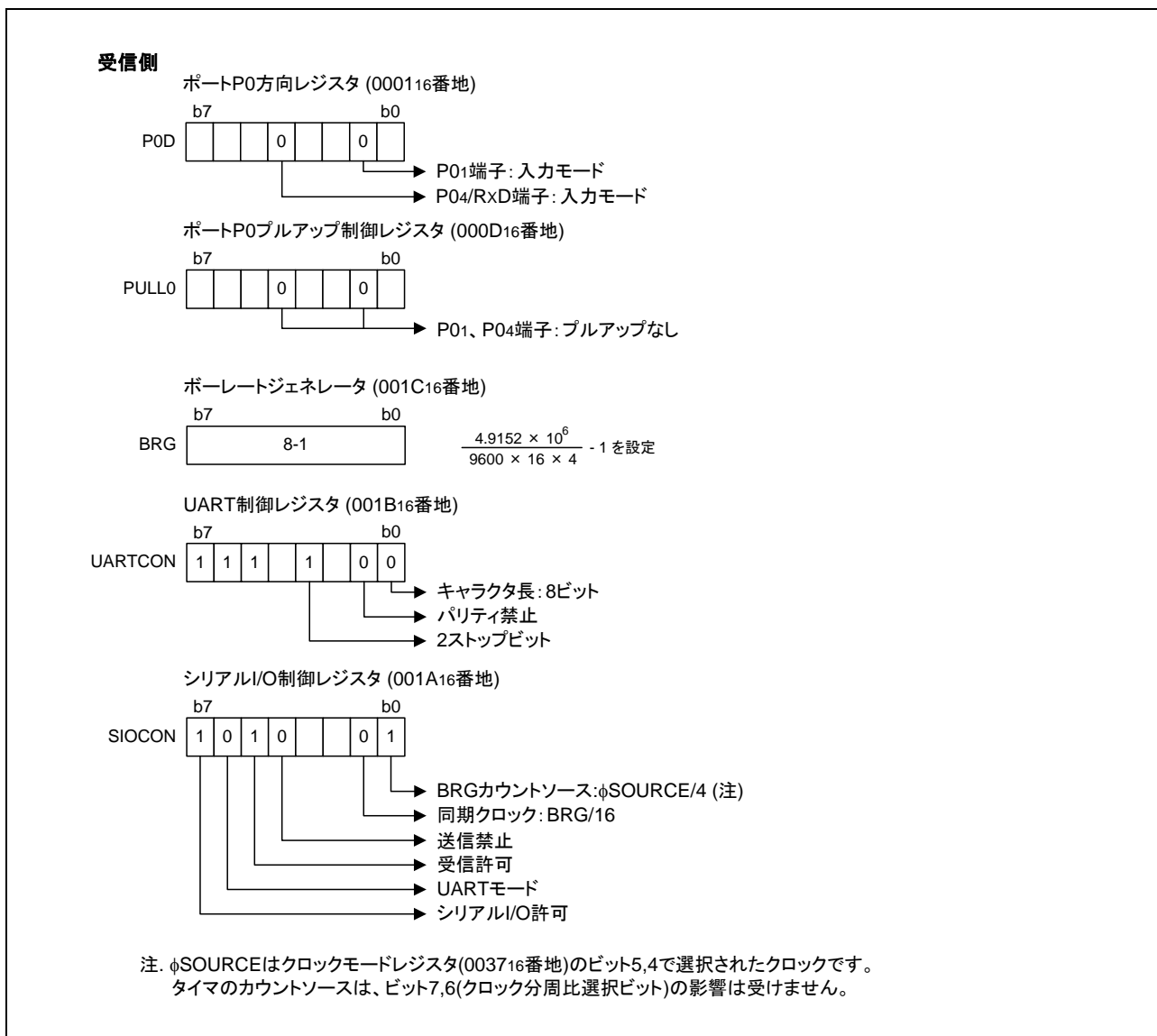
図 3.4 受信側関連レジスタの設定(1)
