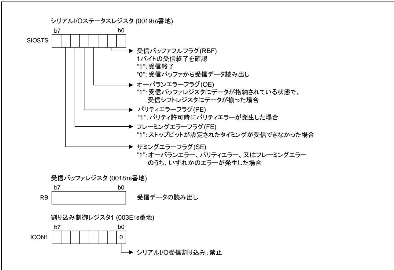
図 3.5 受信側関連レジスタの設定 (2)
