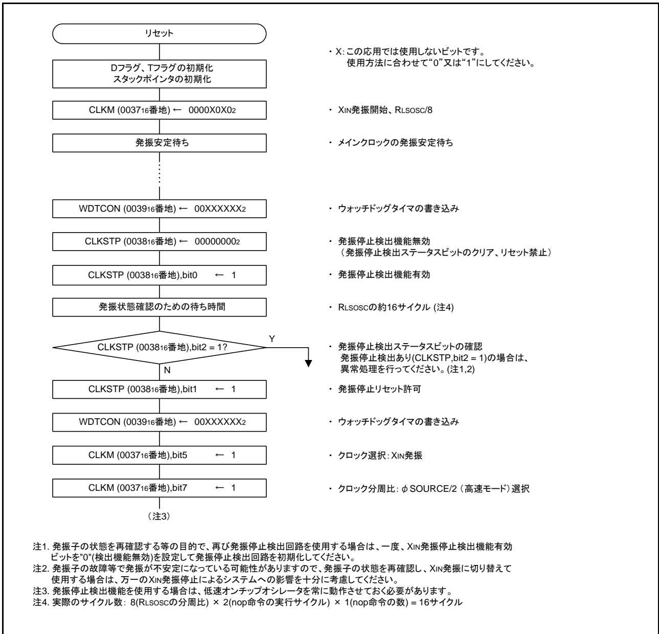
図 3.3 制御手順
