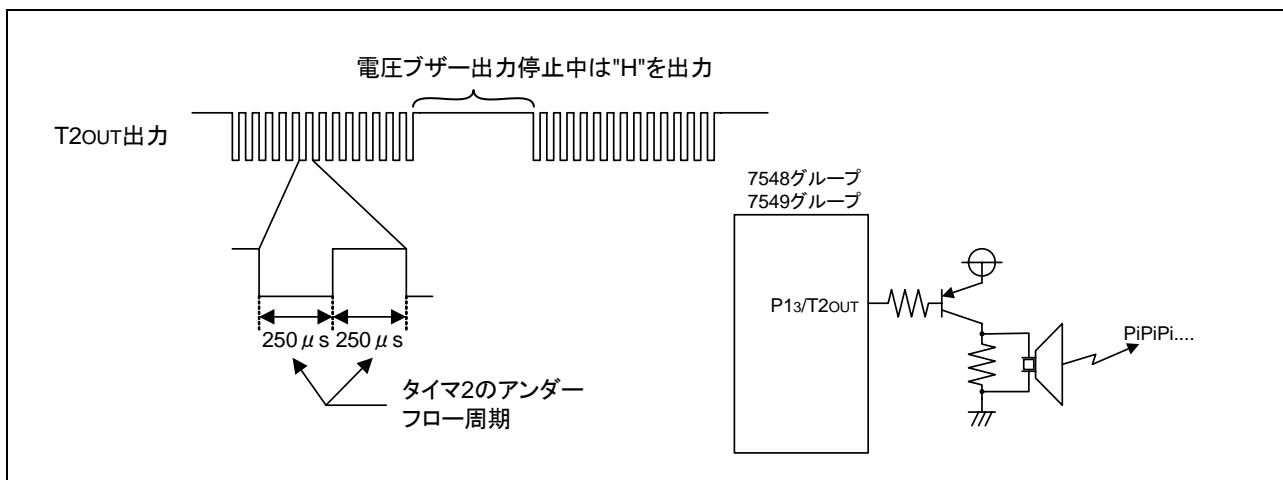
図 3.1 出力波形図及び周辺回路例
