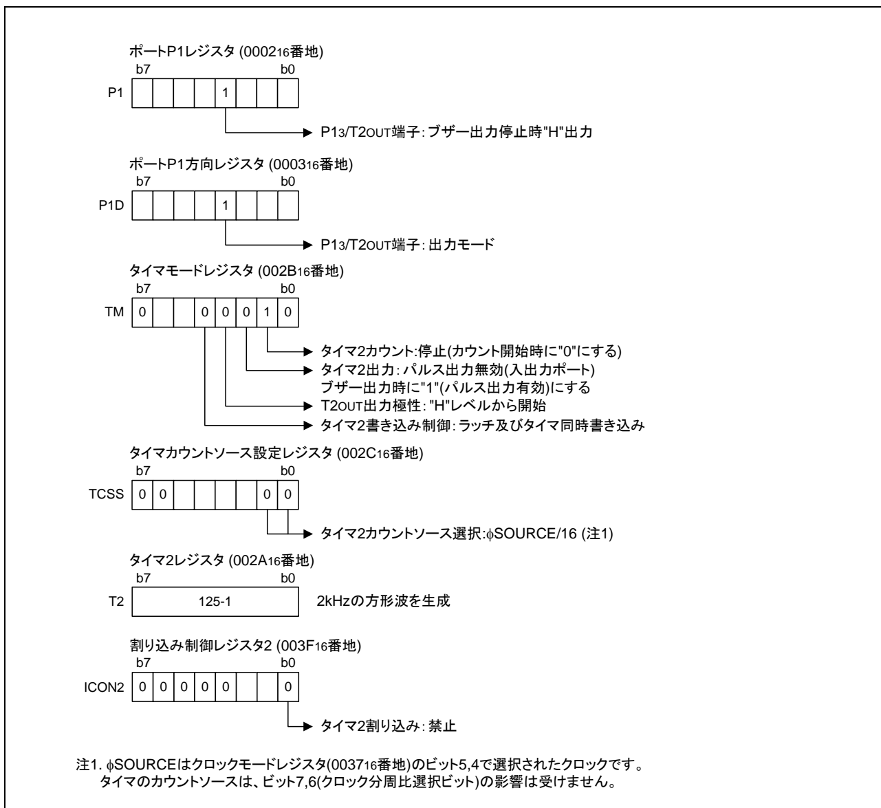
図 3.3 関連レジスタの設定
