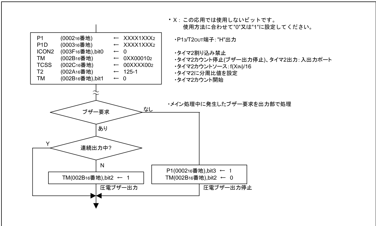
図 3.4 制御手順
