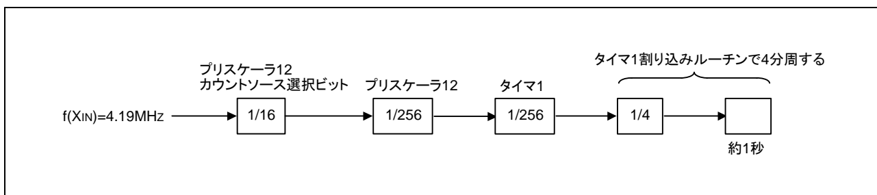
図 3.1 タイマの接続と分周比
