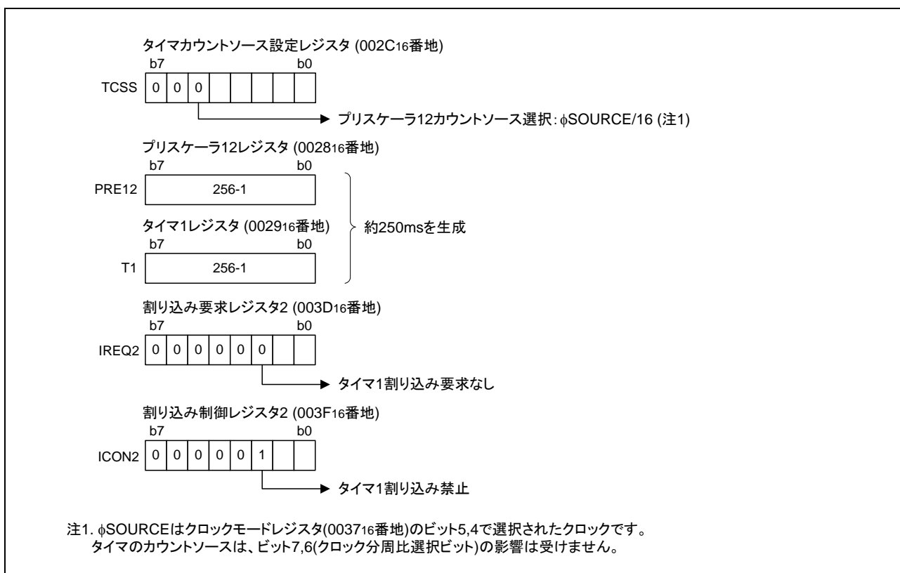
図 3.2 関連レジスタの設定
