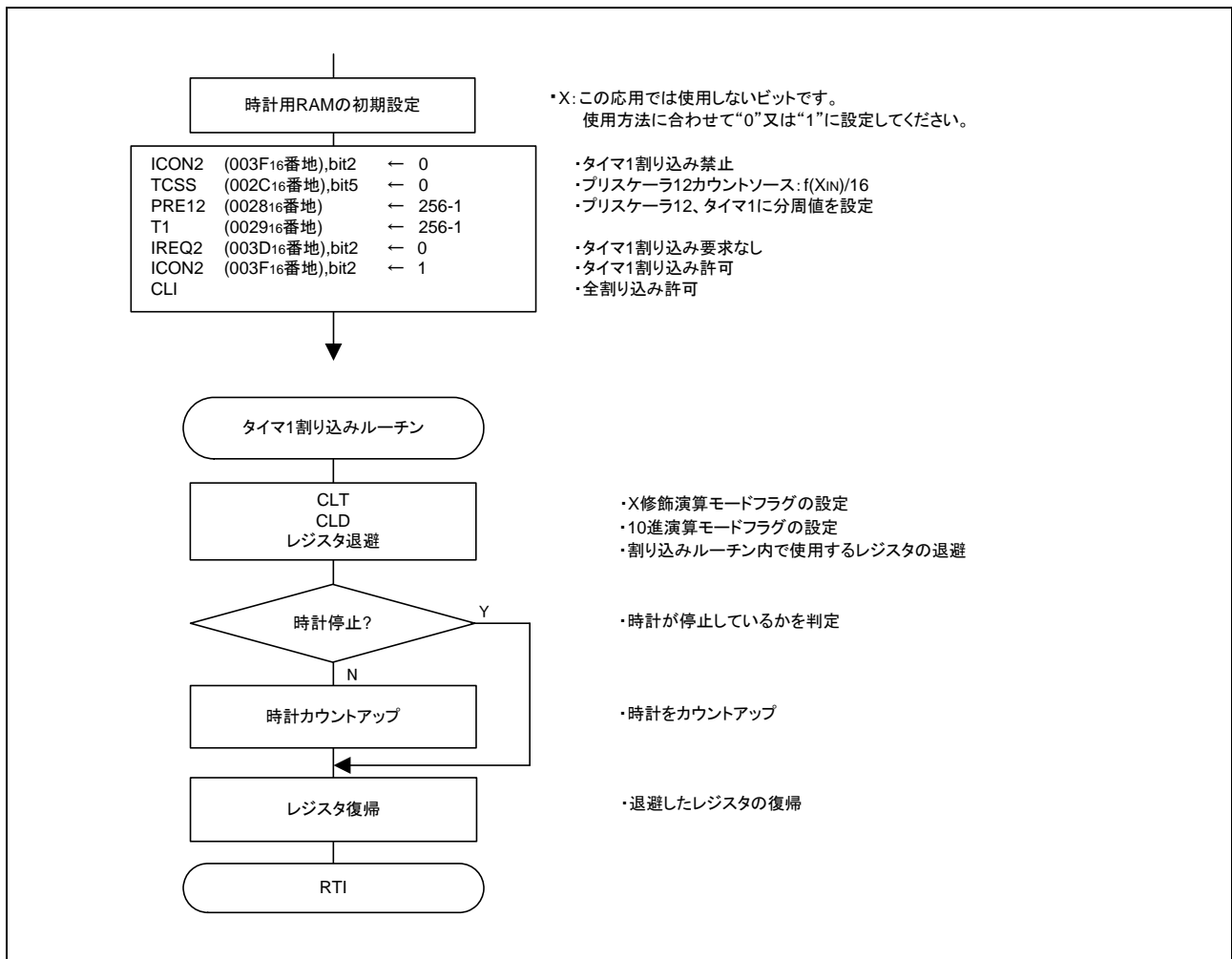
図 3.3 制御手順
