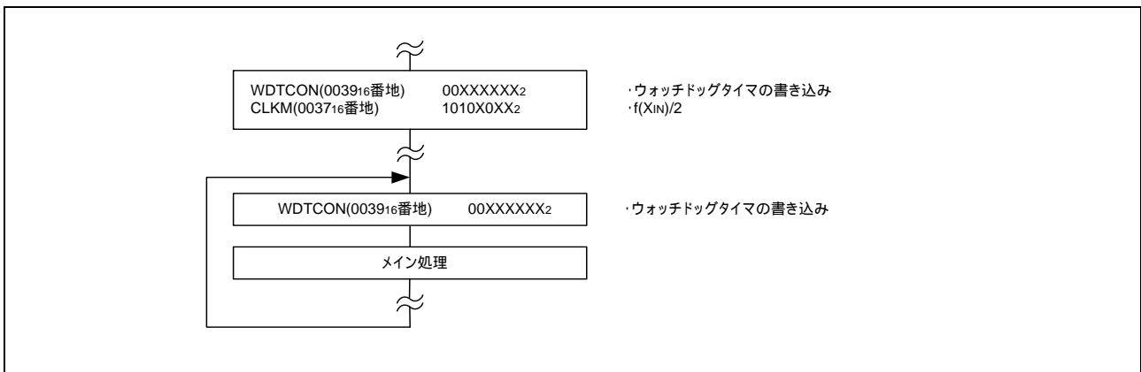
図 3.3 制御手順
