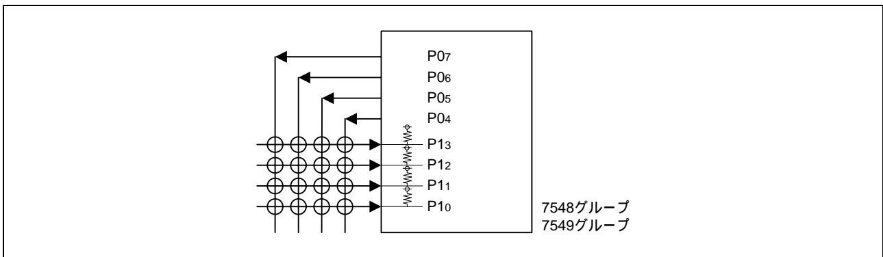
図 3.1 接続図
