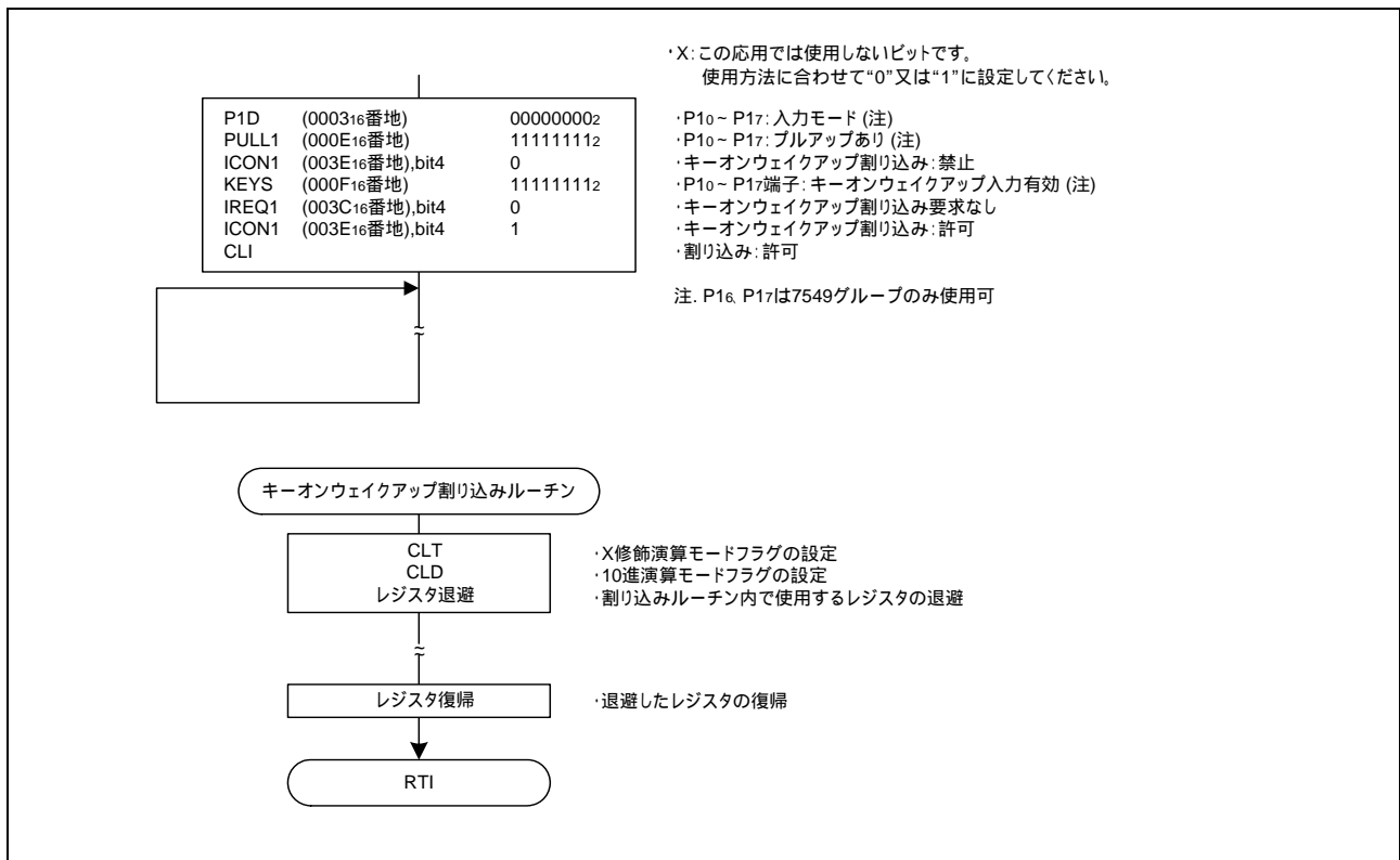
図 3.7 制御手順
