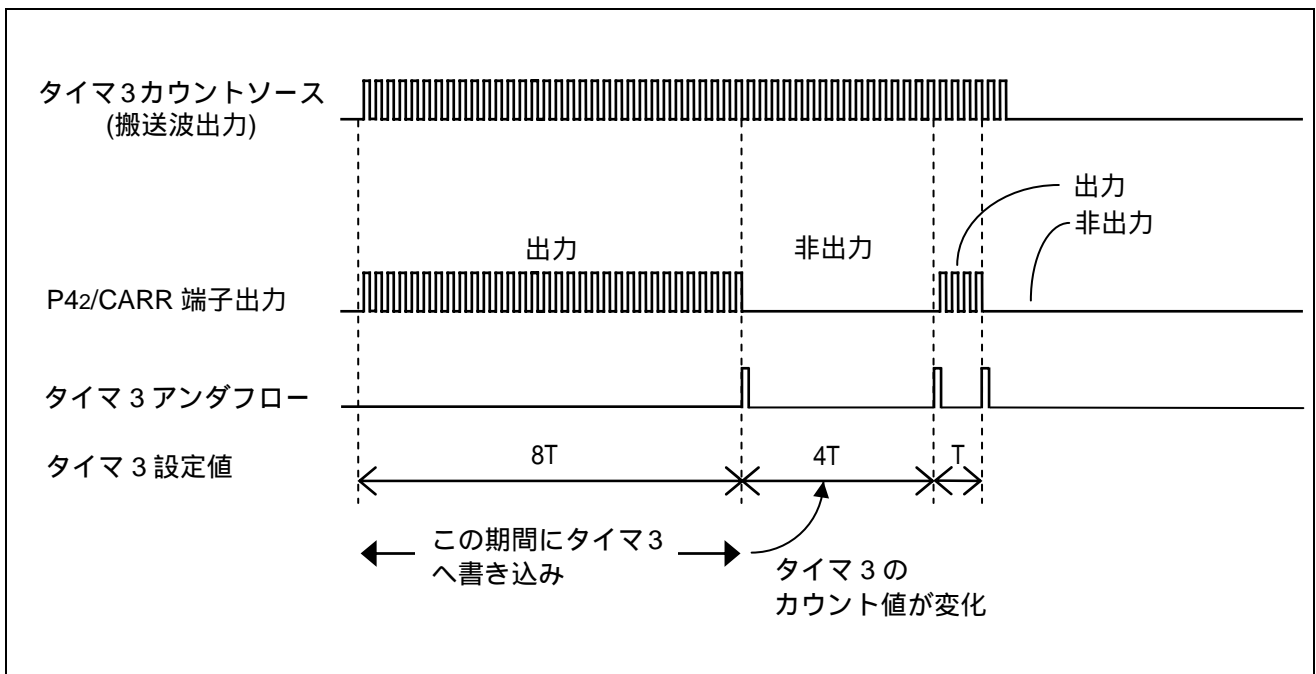
図 1. タイマ 3 による P42/CARR 出力自動制御
