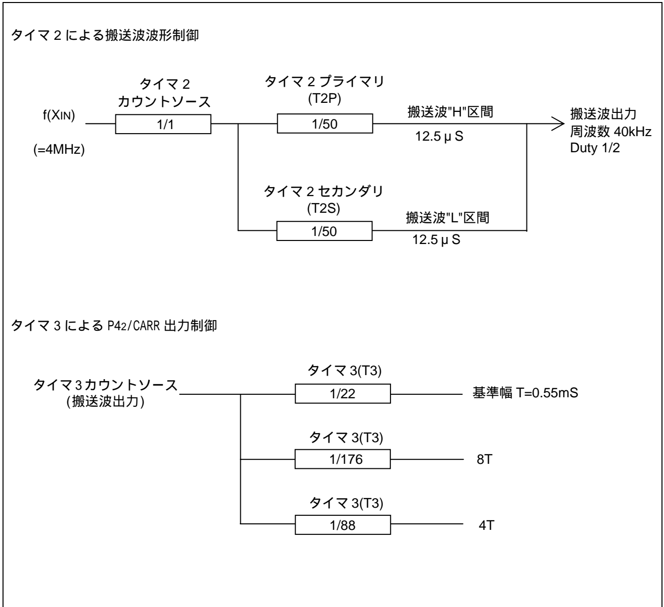
図 2. タイマの接続と分周比
