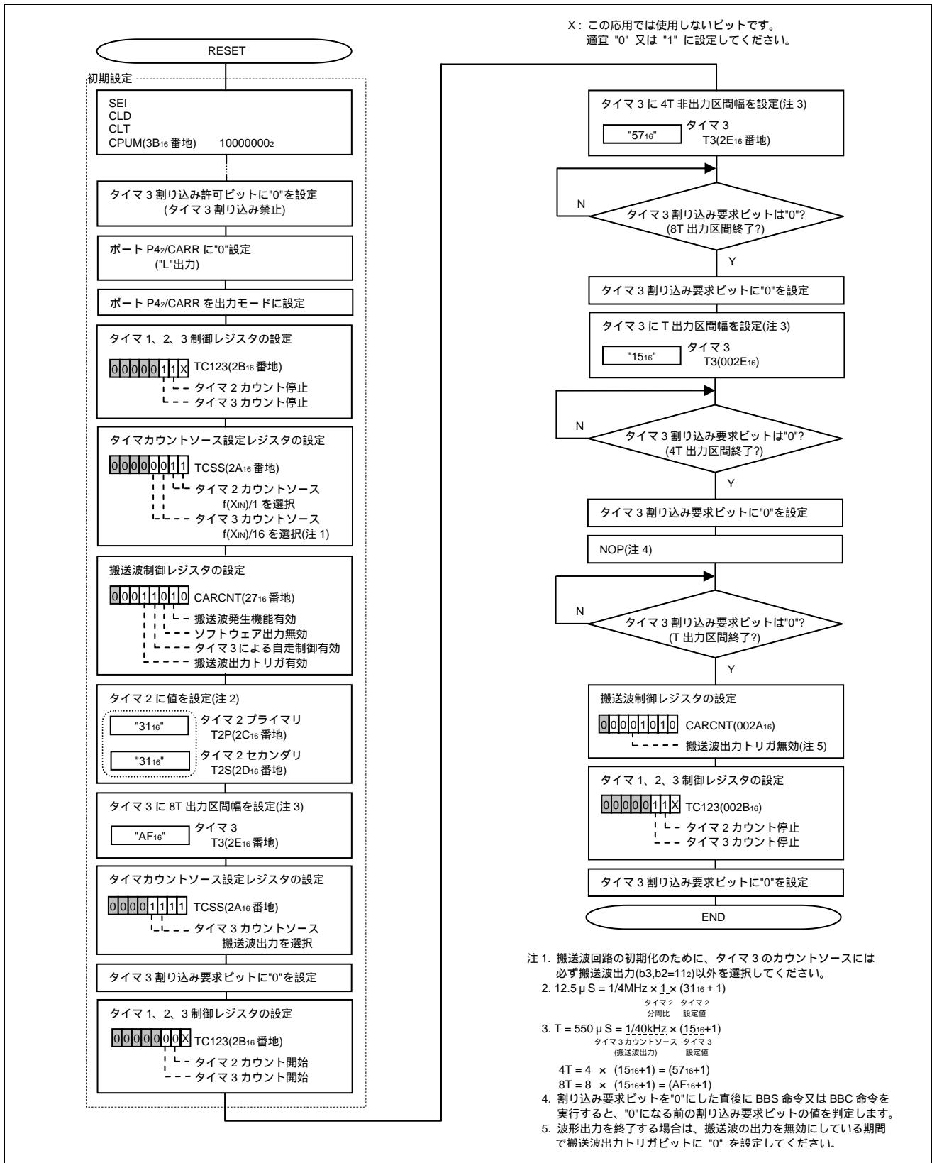
図 3. 制御手順例
