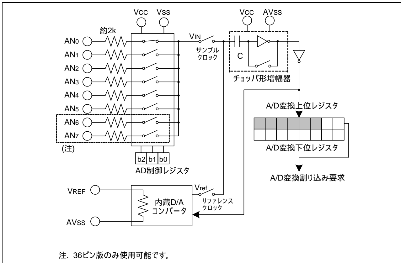
図 3.1 A/Dコンバータ等価回路
