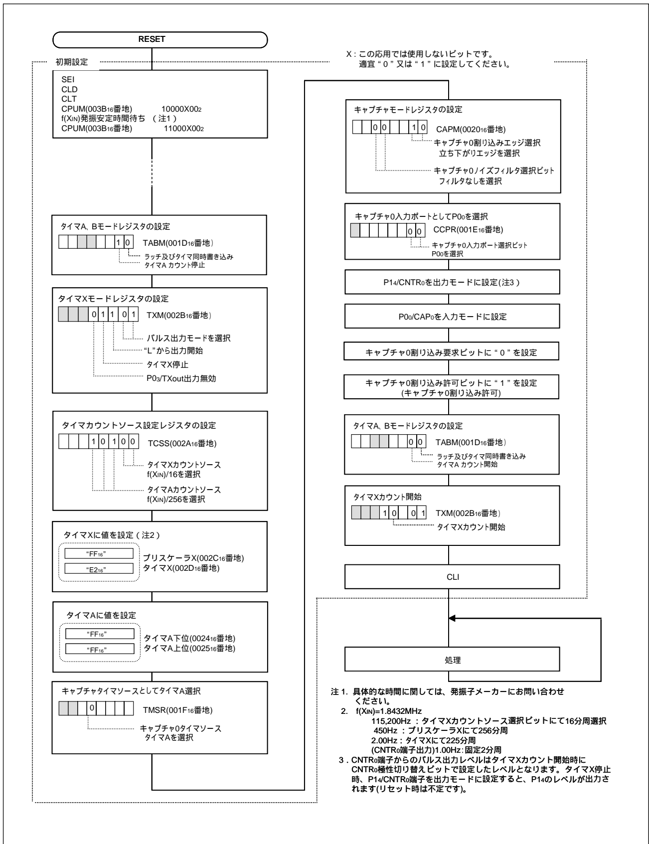
図 5. 制御手順例(1)
