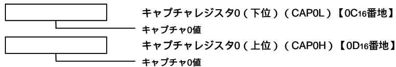
図3. インプットキャプチャの設定方法(3)
