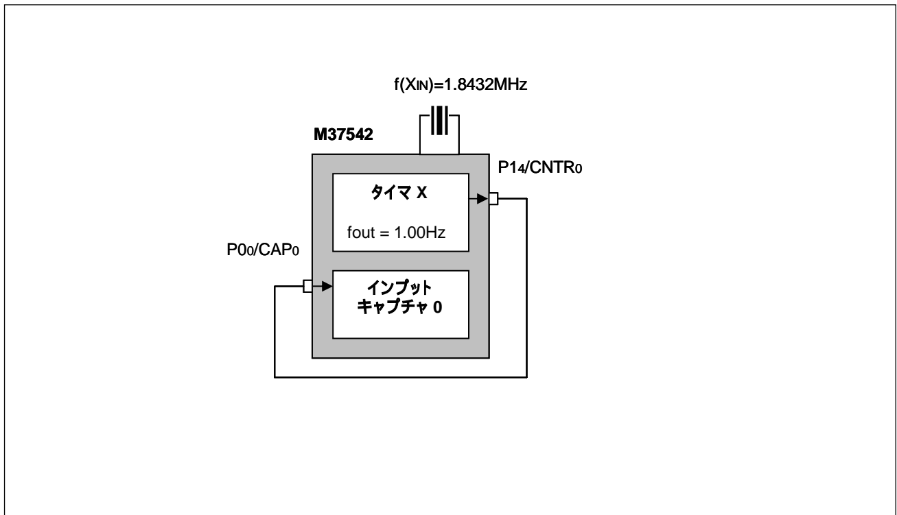
図 4. 周辺回路例
