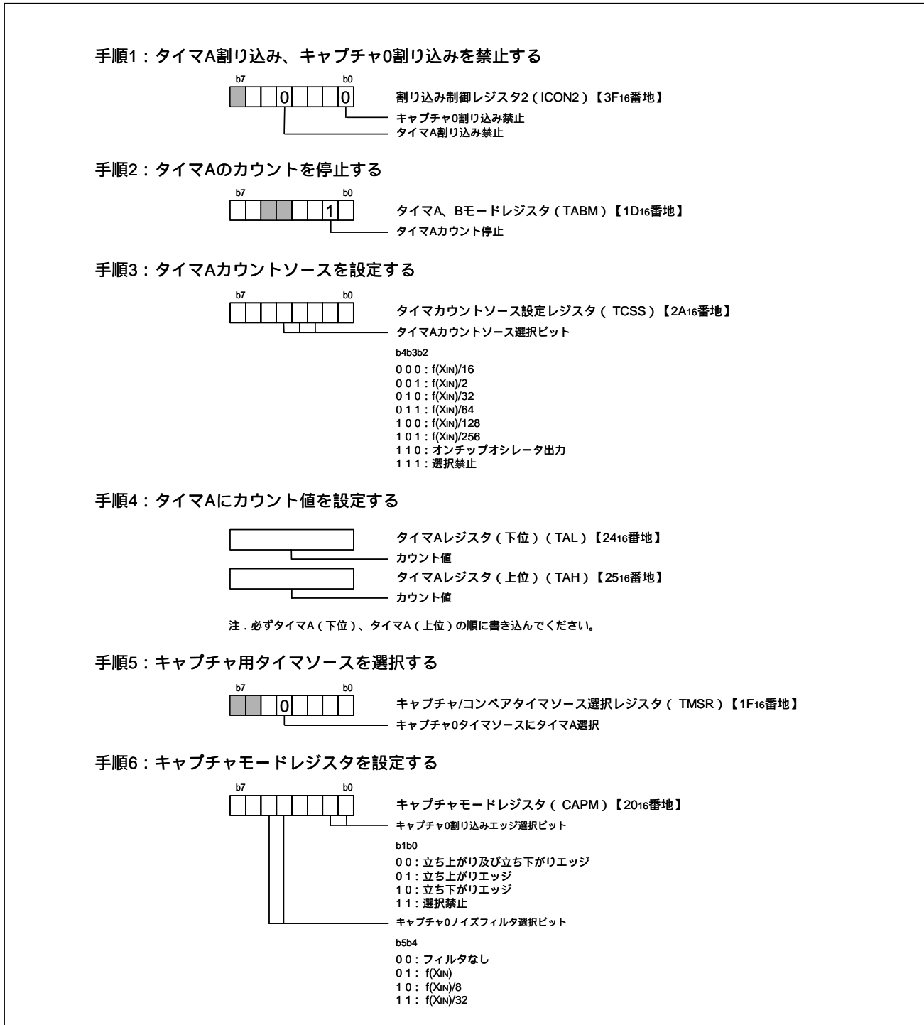
図 1. インプットキャプチャの設定方法(1)
