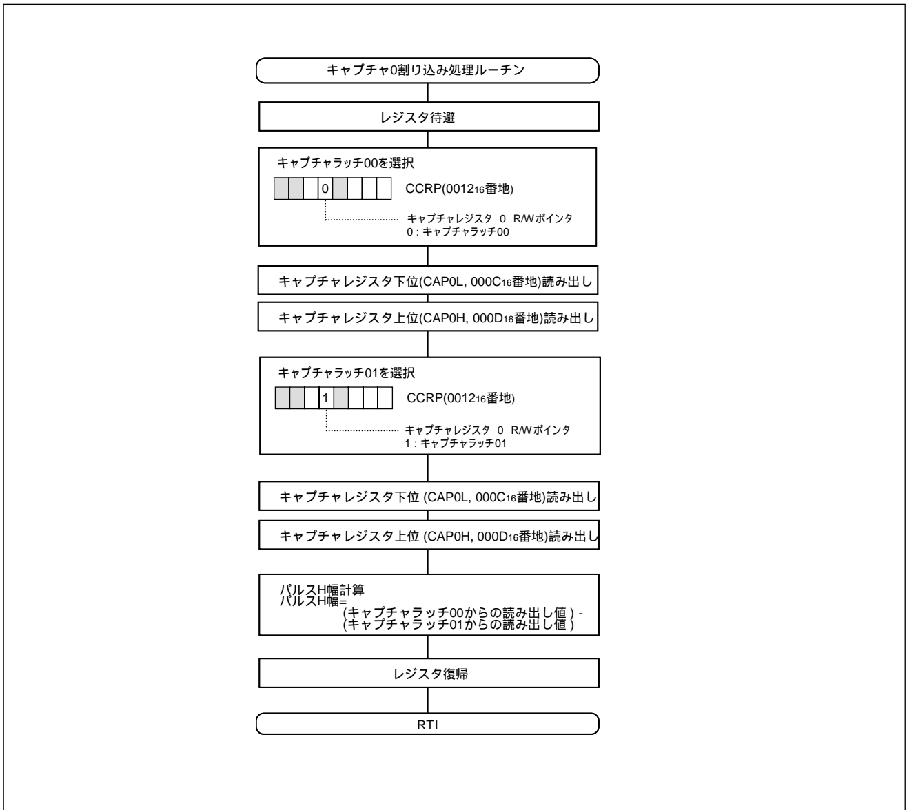
図 6. 制御手順例(2)
