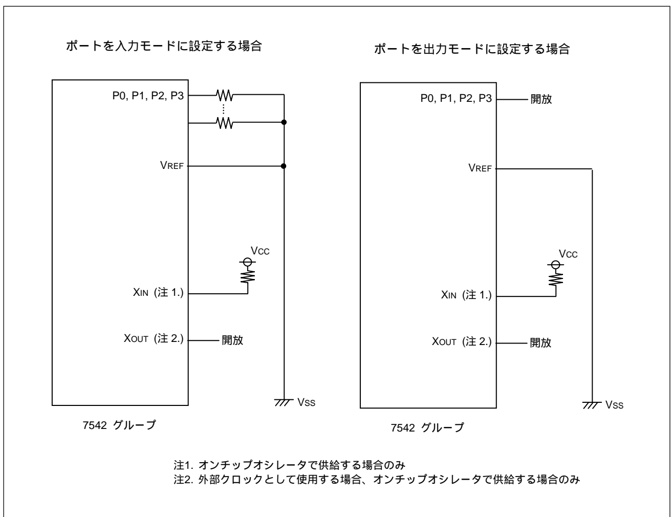
図 3.1 未使用端子の処理例
