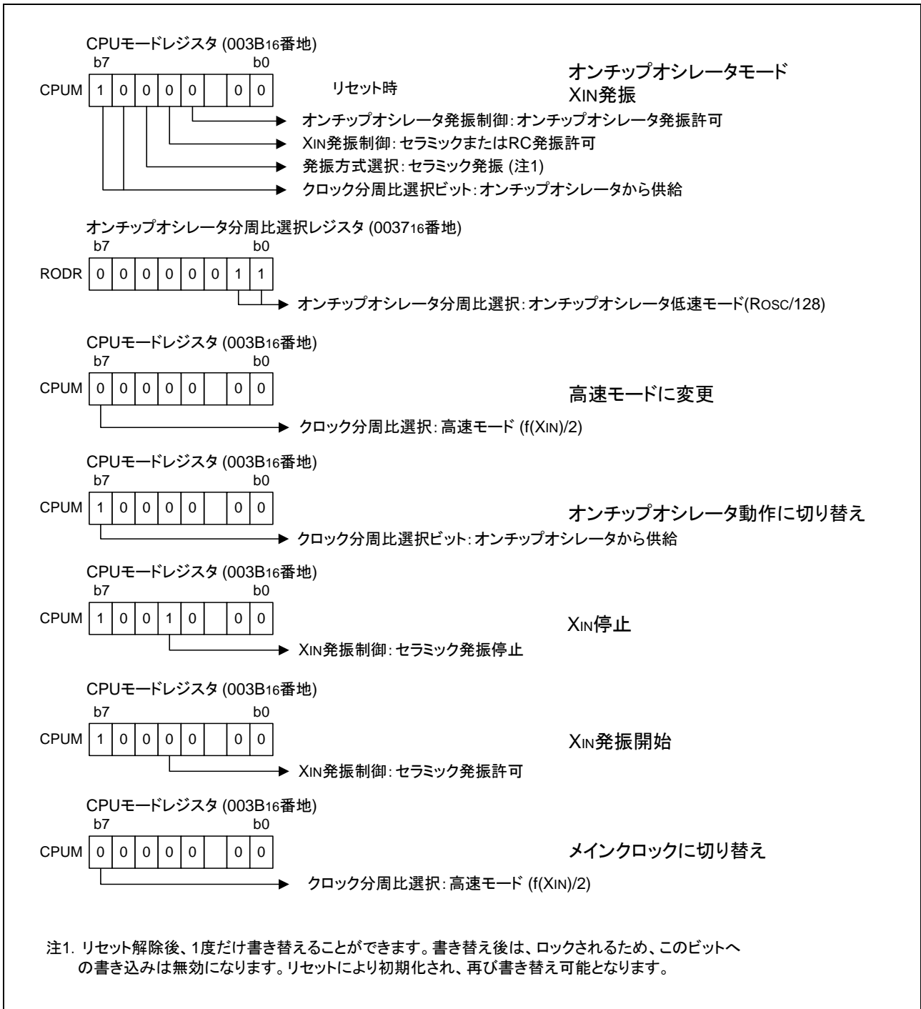
図 3.2 関連レジスタの設定
