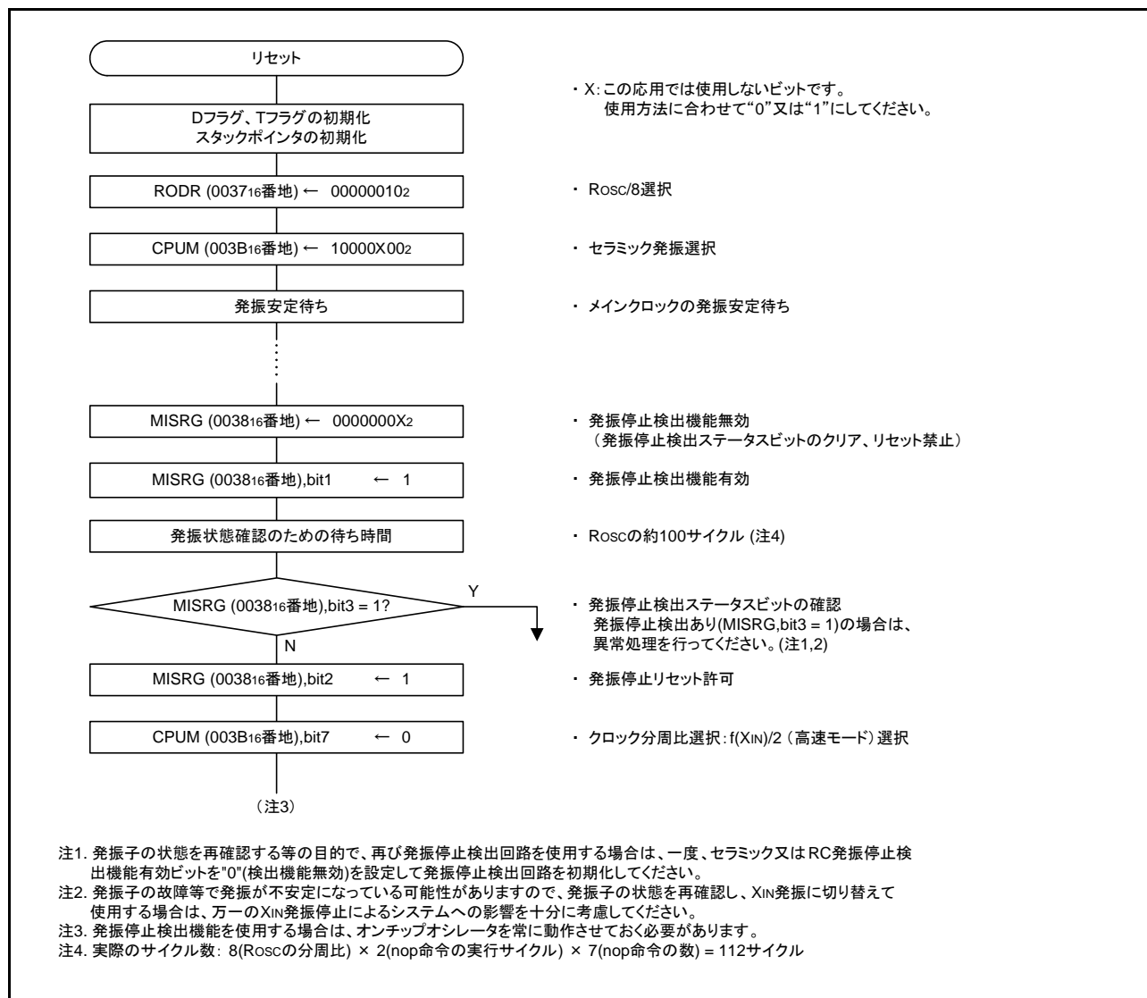
図 3.2 制御手順
