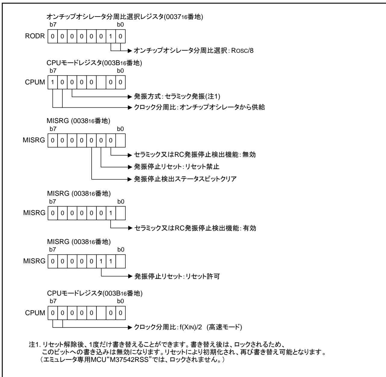
図 3.1 関連レジスタの設定
