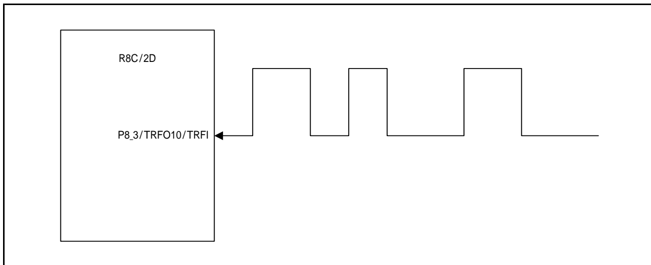
図 3.2 インプットキャプチャ入力
