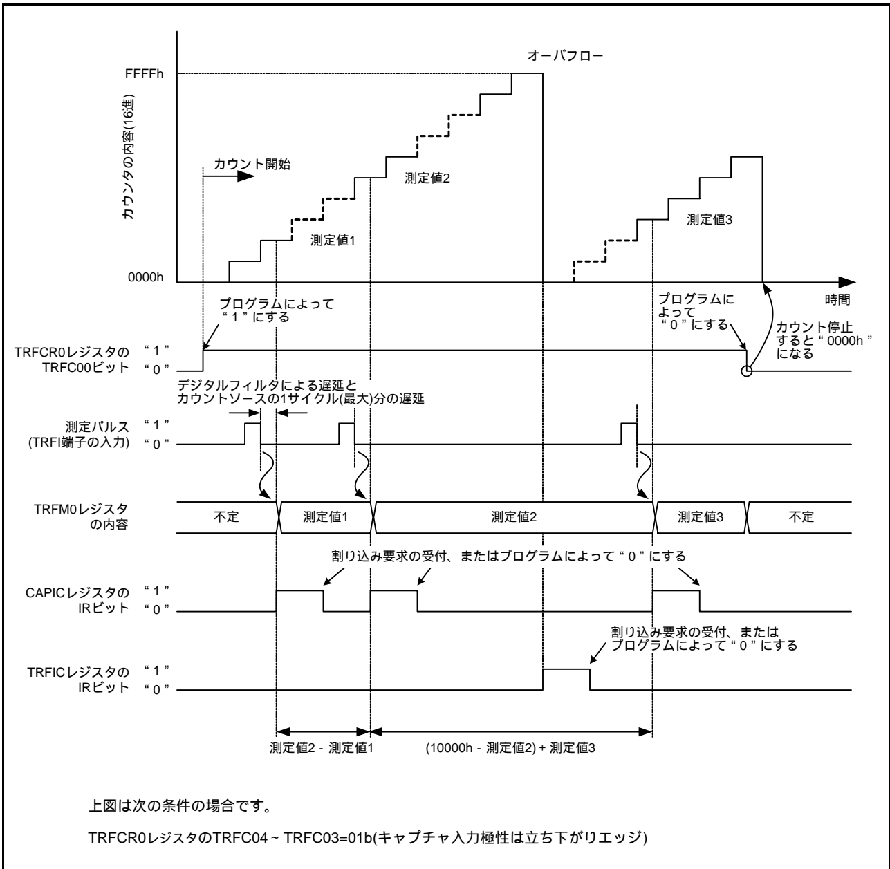
図 3.1 インプットキャプチャモードの動作例
