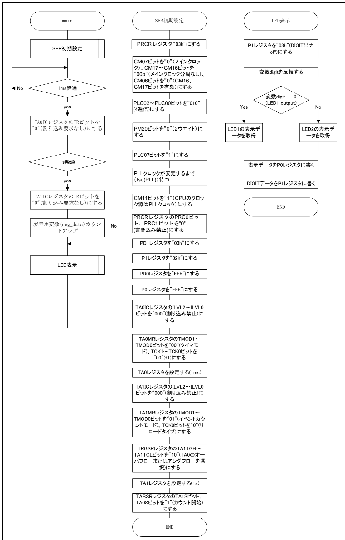
図 3 レジスタ設定フロー図
