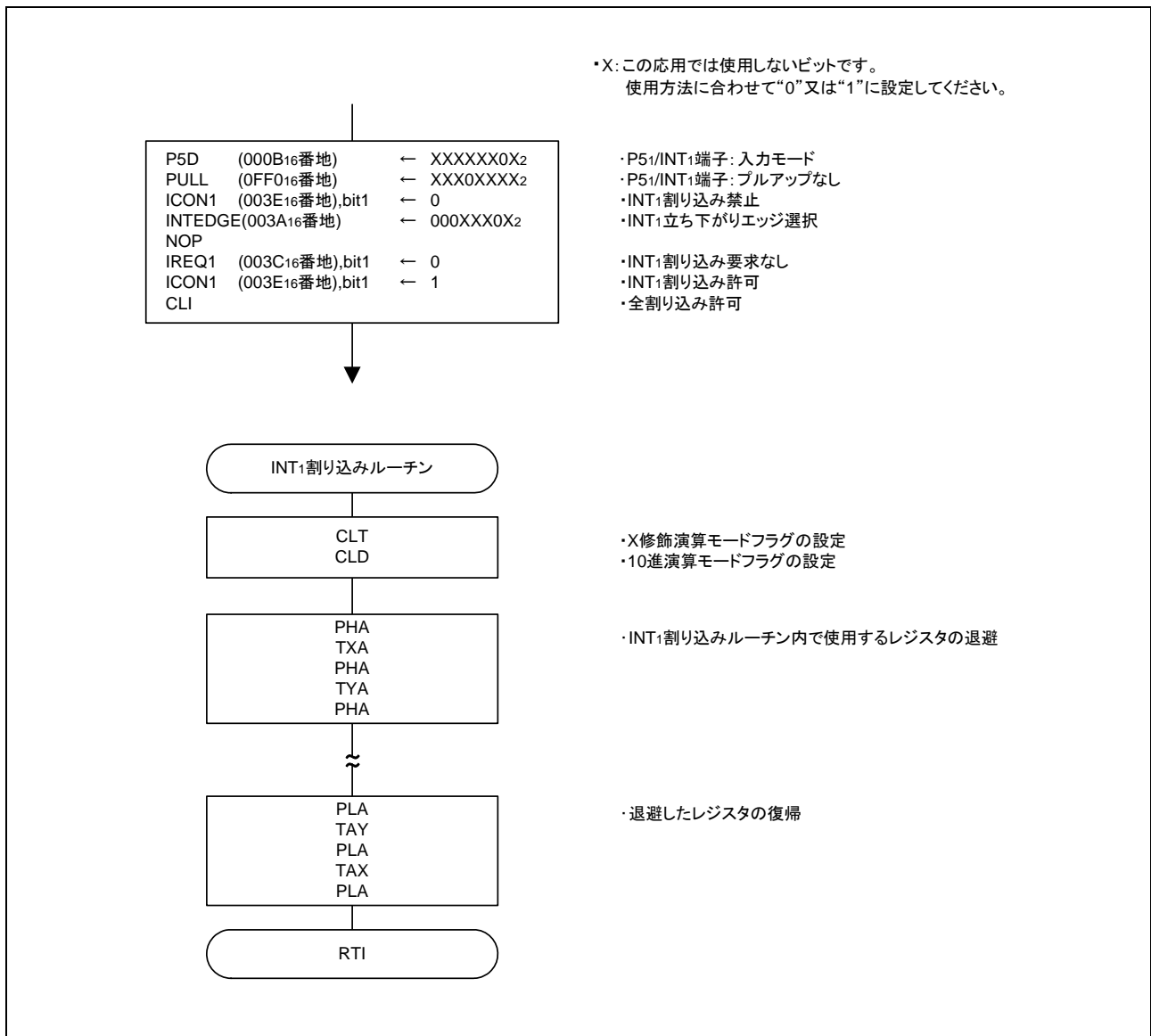
図 3.3 制御手順
