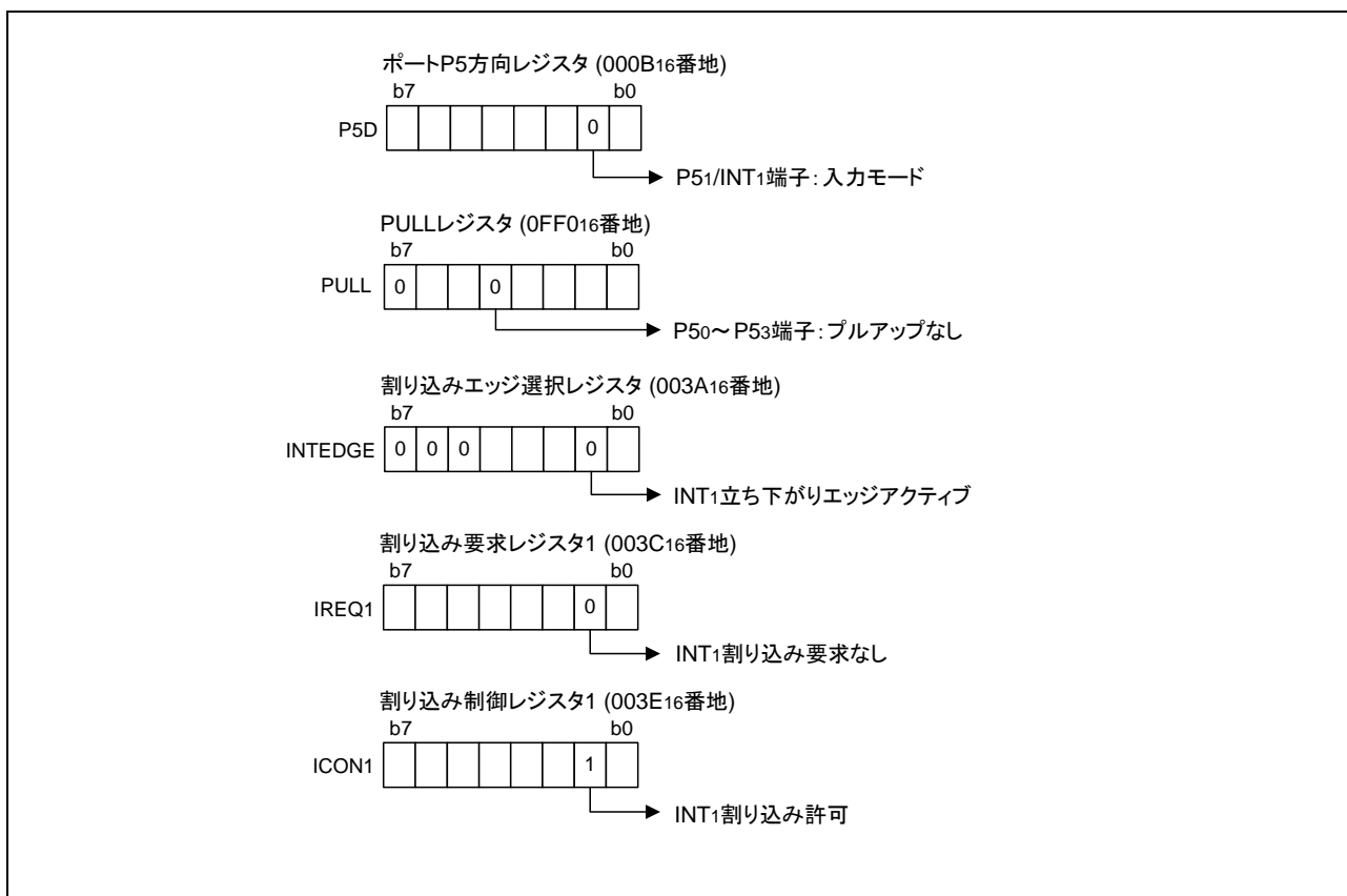
図 3.2 関連レジスタの設定
