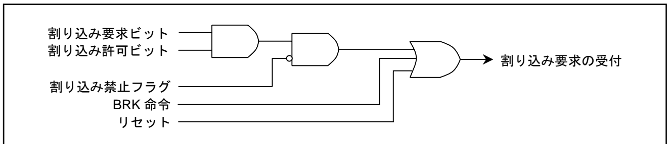
図 3.1 割り込み制御図
