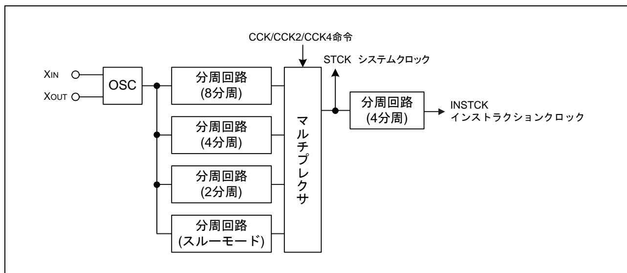
図 3.1 クロック制御回路の構成
