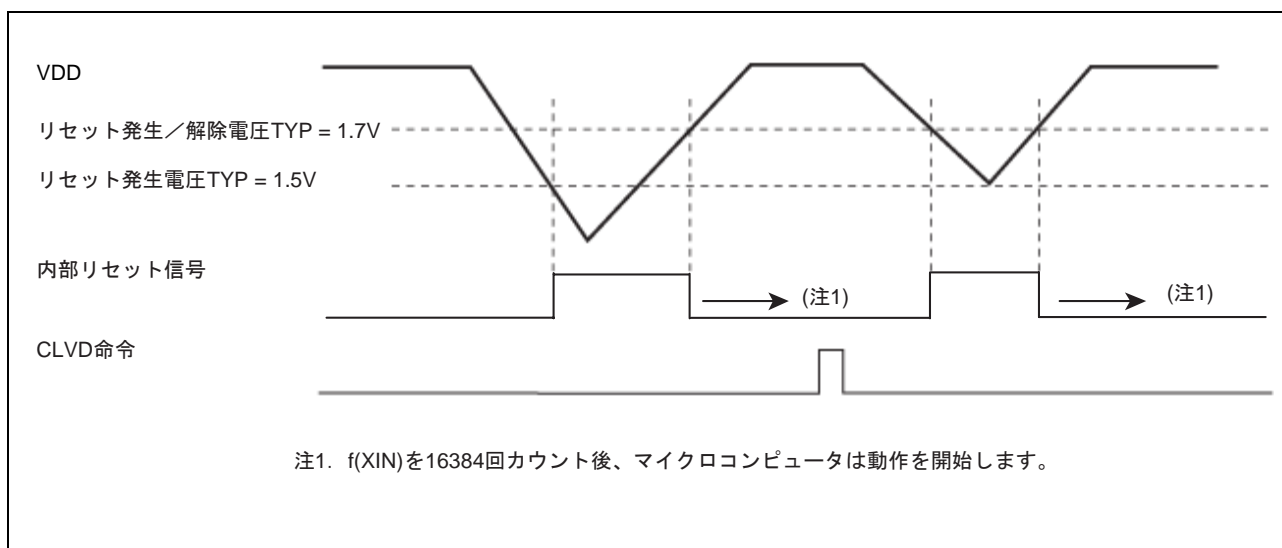
図 3.2 電圧低下検出回路動作波形
