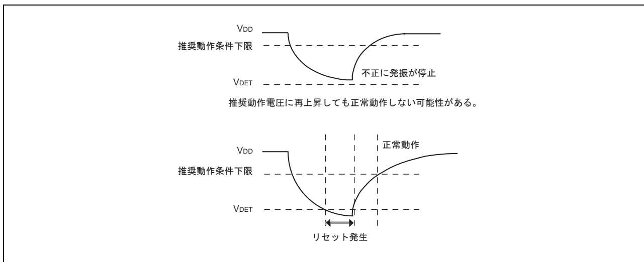
図 3.3 VDDとVDET
