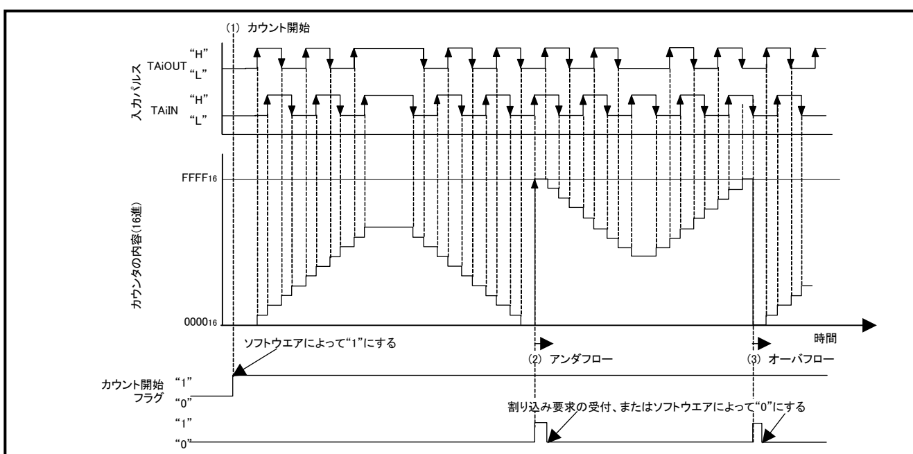
図 1. イベントカウンタモード二相パルス信号処理、4 通倍モード選択時の動作タイミング図
